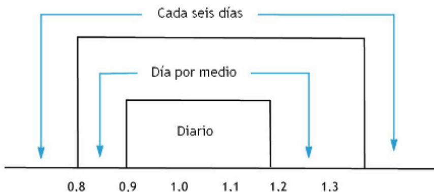
Figura 33. Relación con el límite máximo permisible para 24 horas de PST y PM10 107
