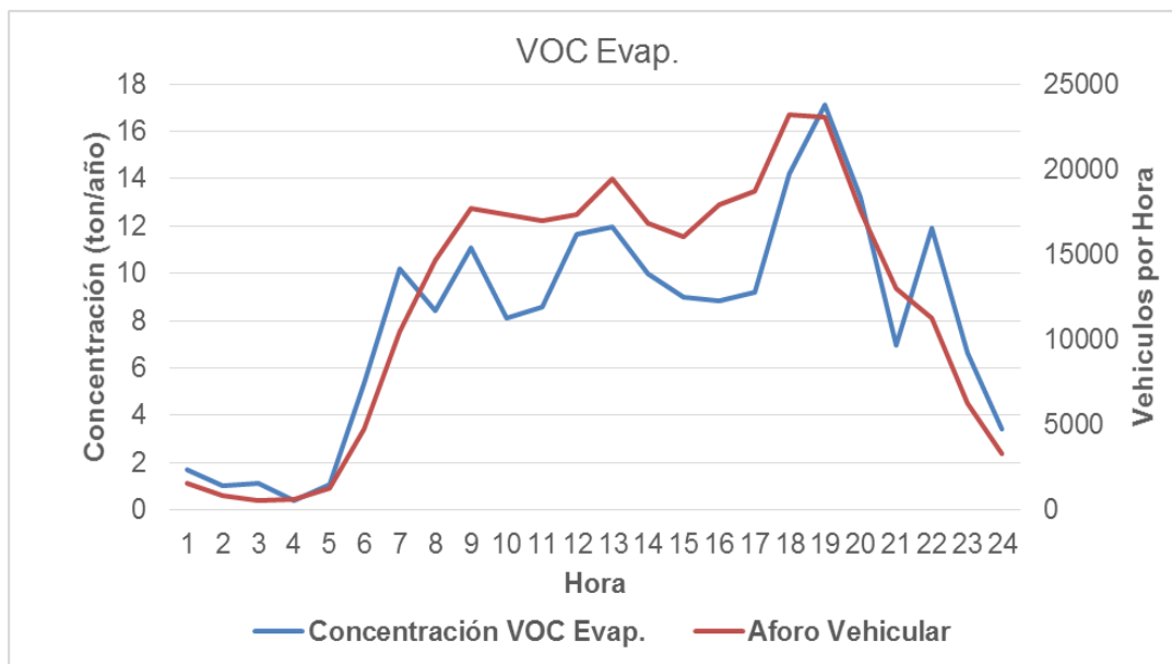
Figura 6.13 Emisión horaria VOC Evap. por fuentes móviles vs aforo vehicular – Cartago. Fuente: K2 Ingeniería S.A.S (estudio actual)
