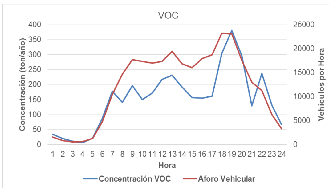
Figura 6.12 Emisión horaria VOC por fuentes móviles vs aforo vehicular – Cartago. Fuente: K2 Ingeniería S.A.S (estudio actual)
