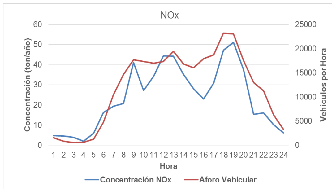
Figura 6.14 Emisión horaria NOx por fuentes móviles vs aforo vehicular – Cartago. Fuente: K2 Ingeniería S.A.S (estudio actual)
