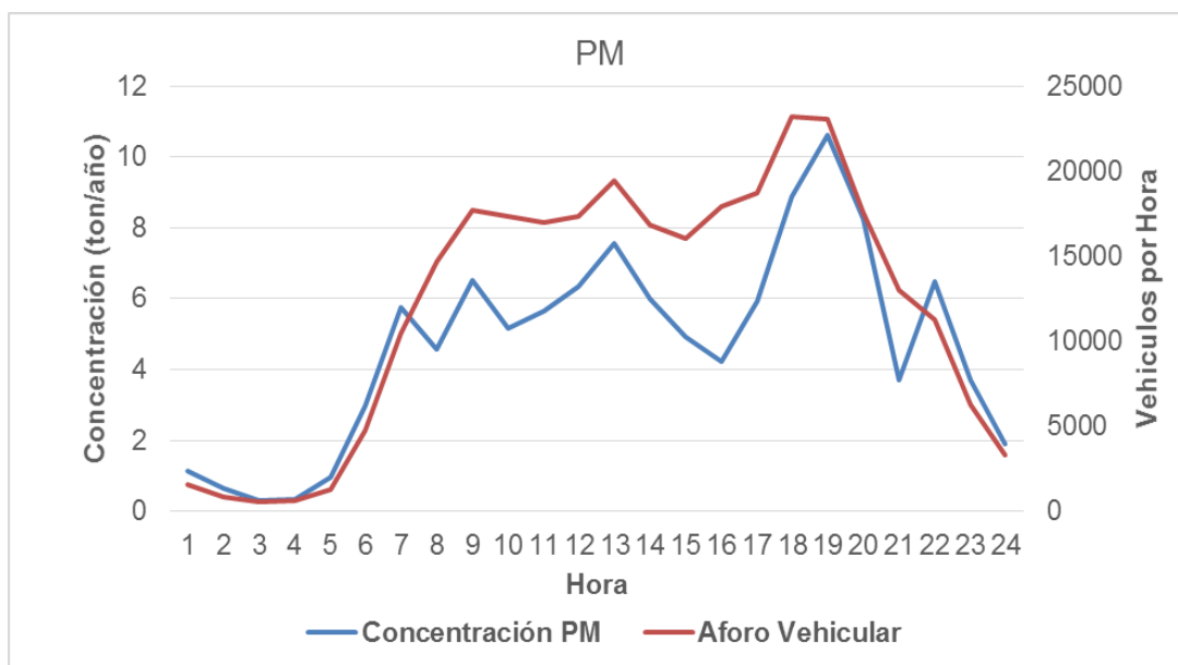
Figura 6.16 Emisión horaria PM por fuentes móviles vs aforo vehicular – Cartago. Fuente: K2 Ingeniería S.A.S (estudio actual)
