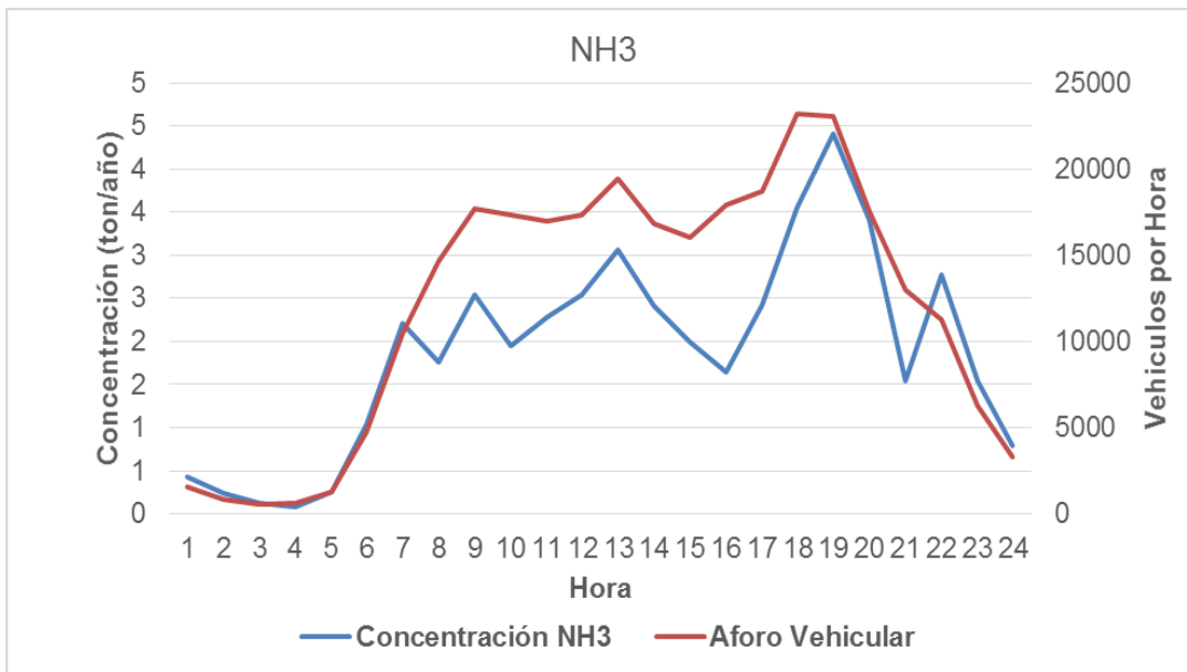
Figura 6.17 Emisión horaria NH 3 por fuentes móviles vs aforo vehicular – Cartago. Fuente: K2 Ingeniería S.A.S (estudio actual)
