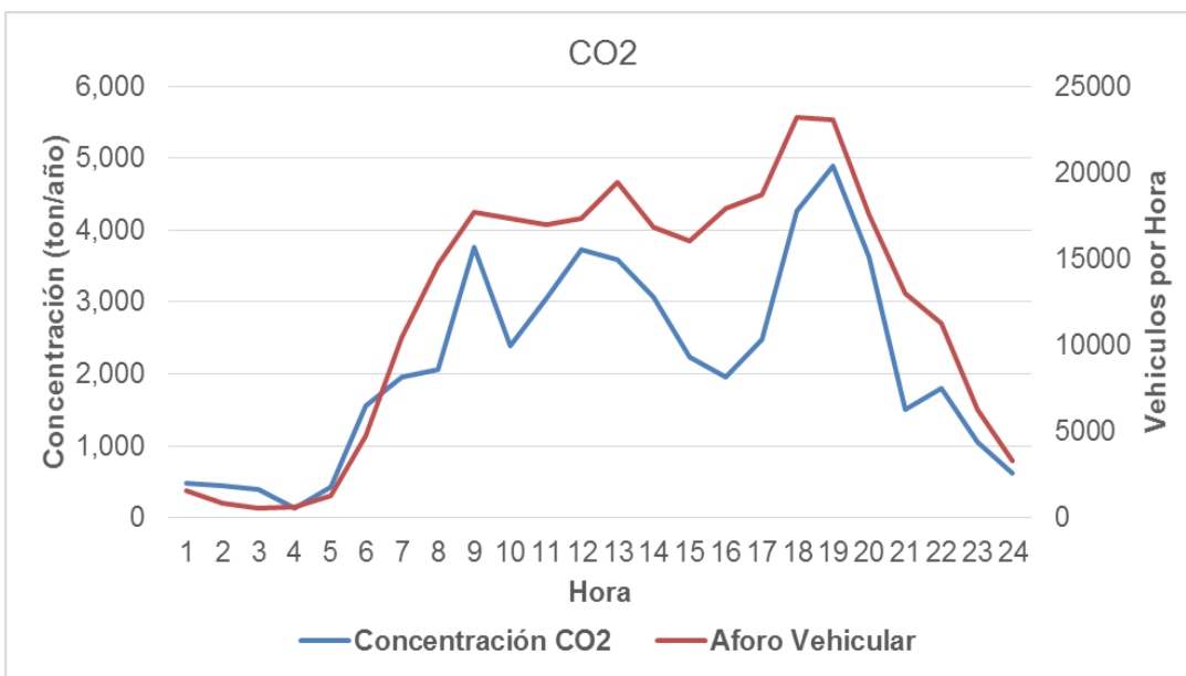
Figura 6.18 Emisión horaria CO 2 por fuentes móviles vs aforo vehicular – Cartago. Fuente: K2 Ingeniería S.A.S (estudio actual)
