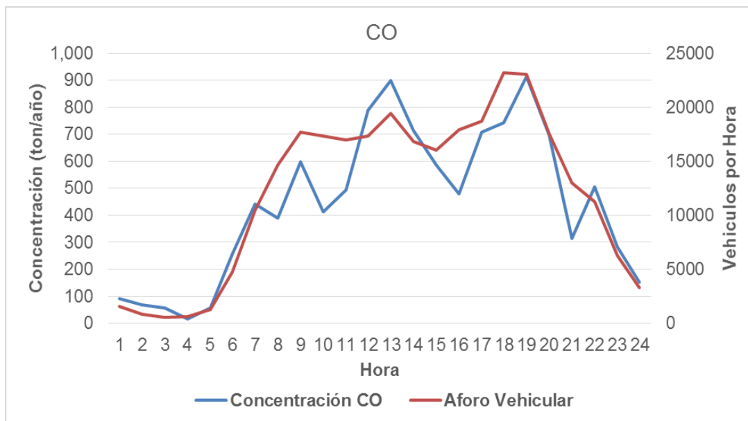
Figura 6.11 Emisión horaria CO por fuentes móviles vs aforo vehicular – Cartago. Fuente: K2 Ingeniería S.A.S (estudio actual)
