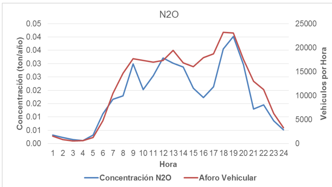
Figura 6.19 Emisión horaria N 2 O por fuentes móviles vs aforo vehicular – Cartago. Fuente: K2 Ingeniería S.A.S (estudio actual)
