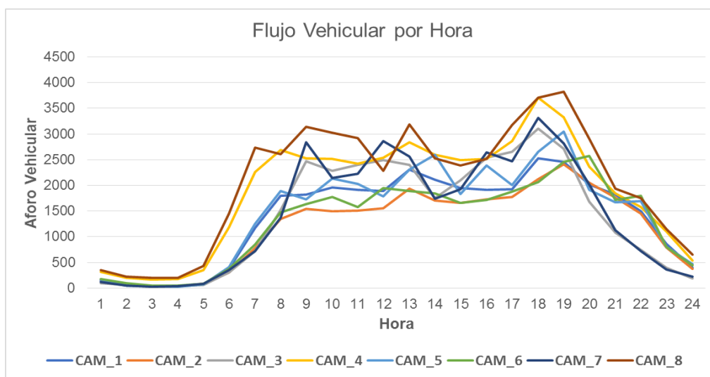
Figura 5.8 Flujo vehicular por hora en jornada ordinaria - Cartago
