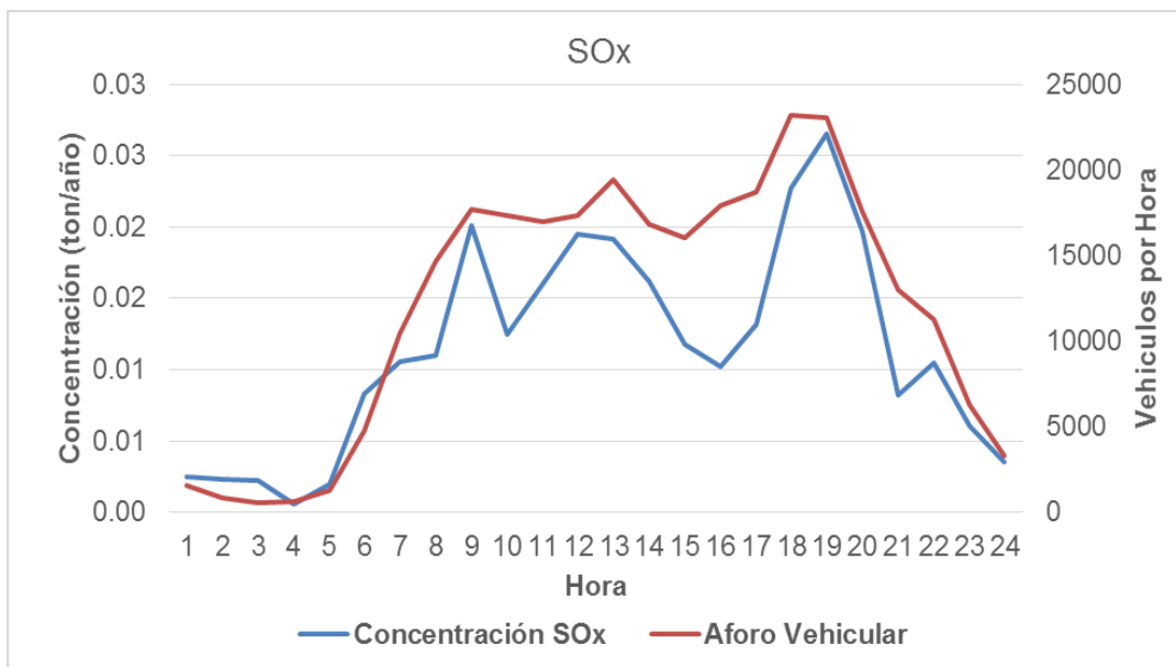
Figura 6.15 Emisión horaria SOx por fuentes móviles vs aforo vehicular – Cartago. Fuente: K2 Ingeniería S.A.S (estudio actual)
