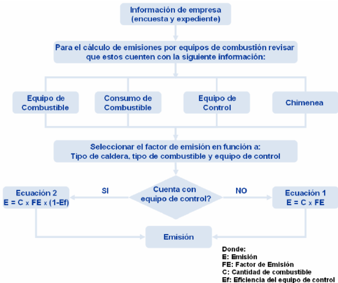
Figura 5.1 Algoritmo para el cálculo de emisiones por combustión Fuente: MADS (Manual de Inventario de Fuentes Puntuales)
