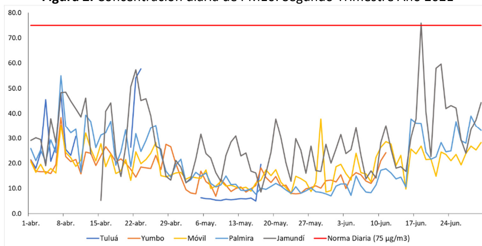
Figura 2. Concentración diaria de PM10. Segundo Trimestre Año 2021
