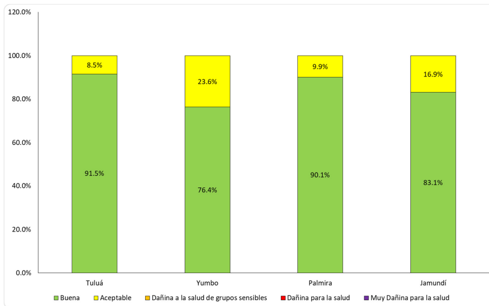
Figura 9. ICA de las concentraciones diarias promedio de PM2.5. Segundo Trimestre de 2020
