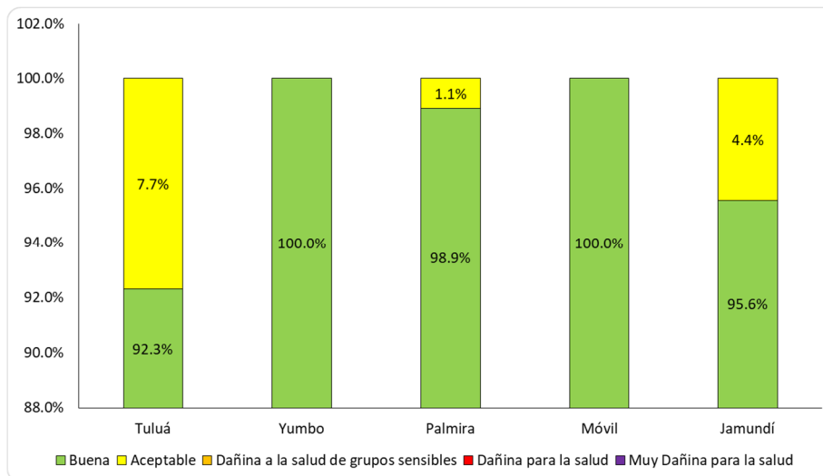
Figura 4. ICA de las concentraciones diarias promedio de PM10. Segundo Trimestre Año 2021
