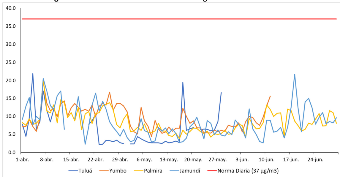
Figura 3. Concentración diaria de PM2.5. Segundo Trimestre Año 2021
