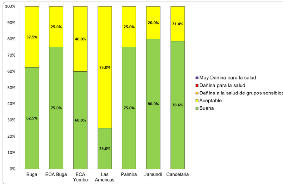
Figura 9. ICA de las concentraciones diarias promedio de PM2.5. Febrero de 2022.
