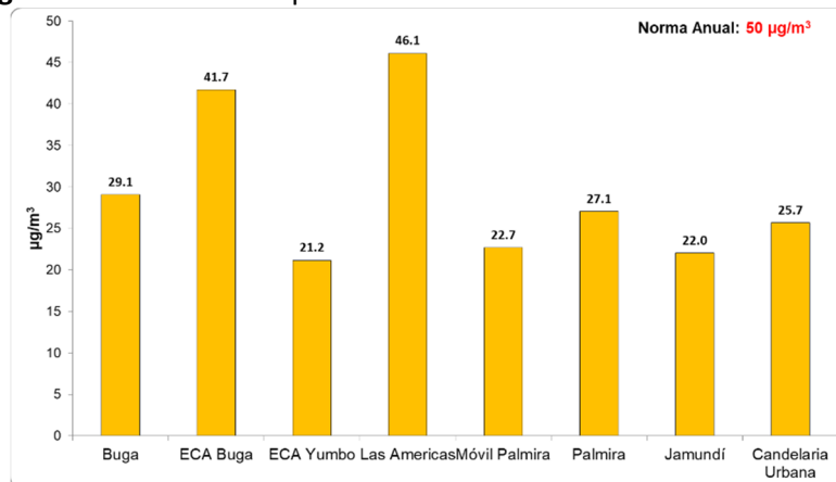
Figura 2. Concentración promedio mensual de PM10. Febrero de 2022
