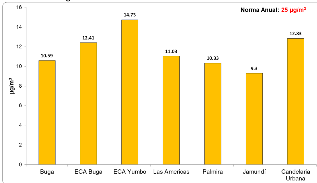
Figura 3. Concentración diaria de PM2.5. Febrero de 2022
