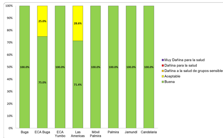
Figura 4. ICA de las concentraciones diarias promedio de PM10. Febrero de 2022
