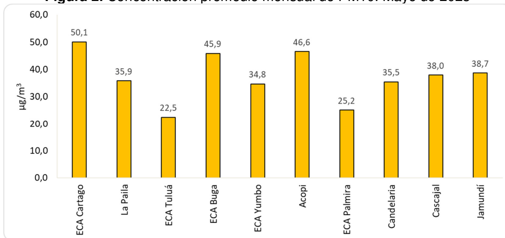
Figura 2. Concentración promedio mensual de PM10. Mayo de 2023
