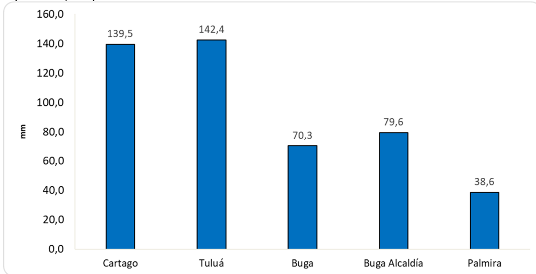
Figura 5. Precipitación acumulada en mayo de 2023.
