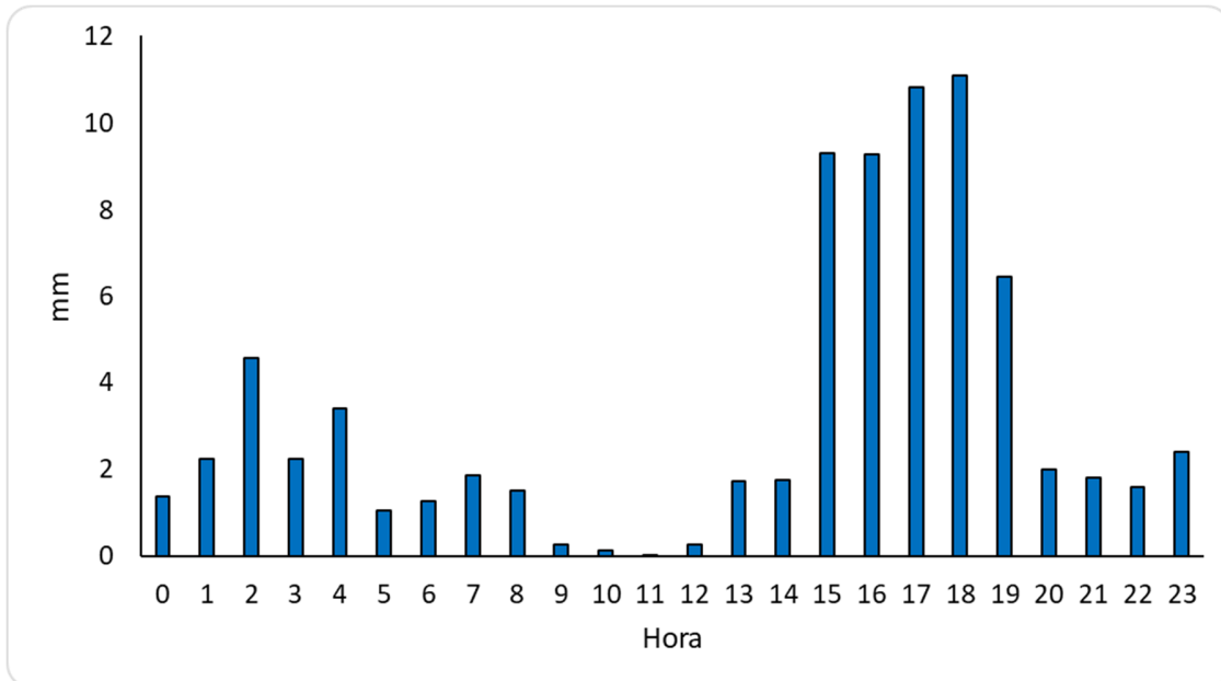
Figura 6. Precipitación acumulada horaria. Mayo de 2023.
