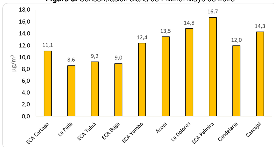
Figura 3. Concentración diaria de PM2.5. Mayo de 2023
