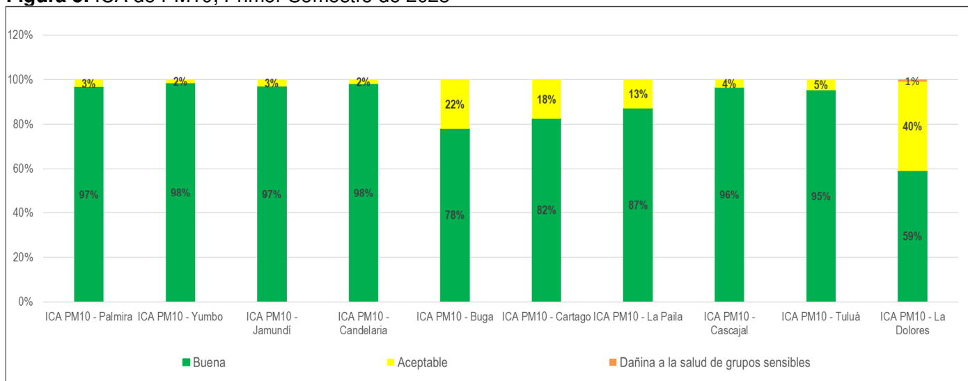
Figura 5. ICA de PM10, Primer Semestre de 2023
