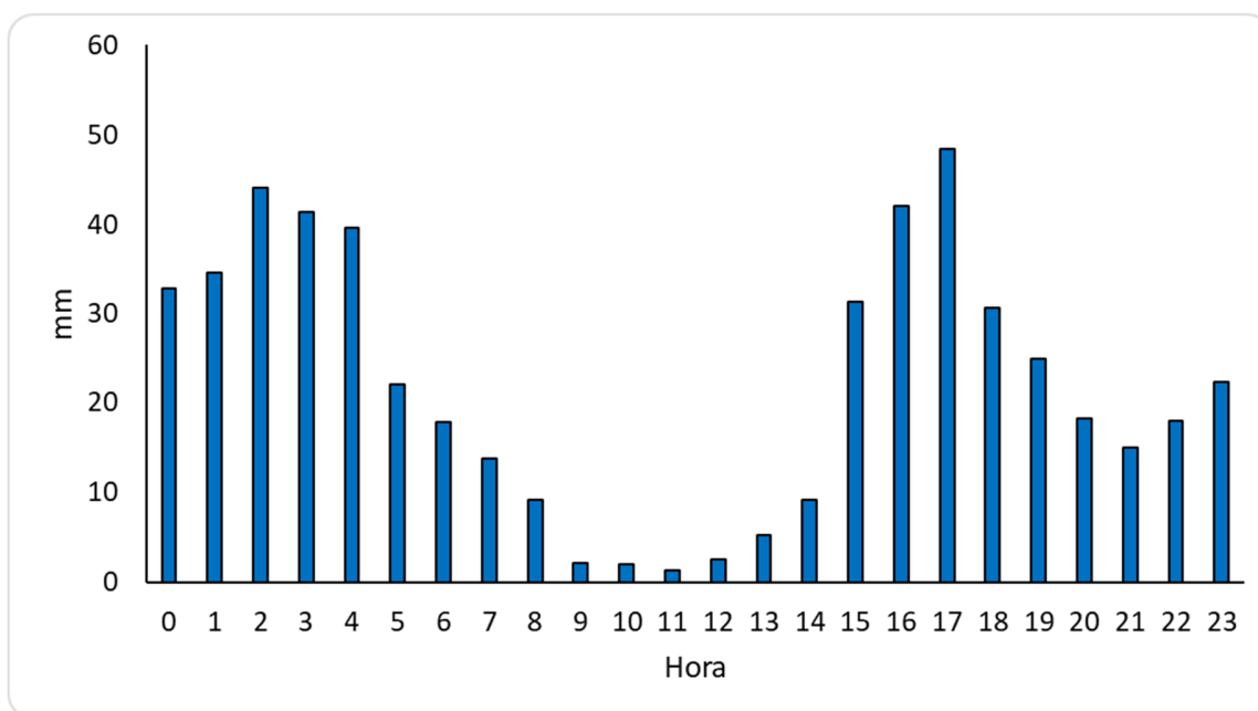
Figura 6. Precipitación acumulada horaria. Primer Semestre de 2023.
