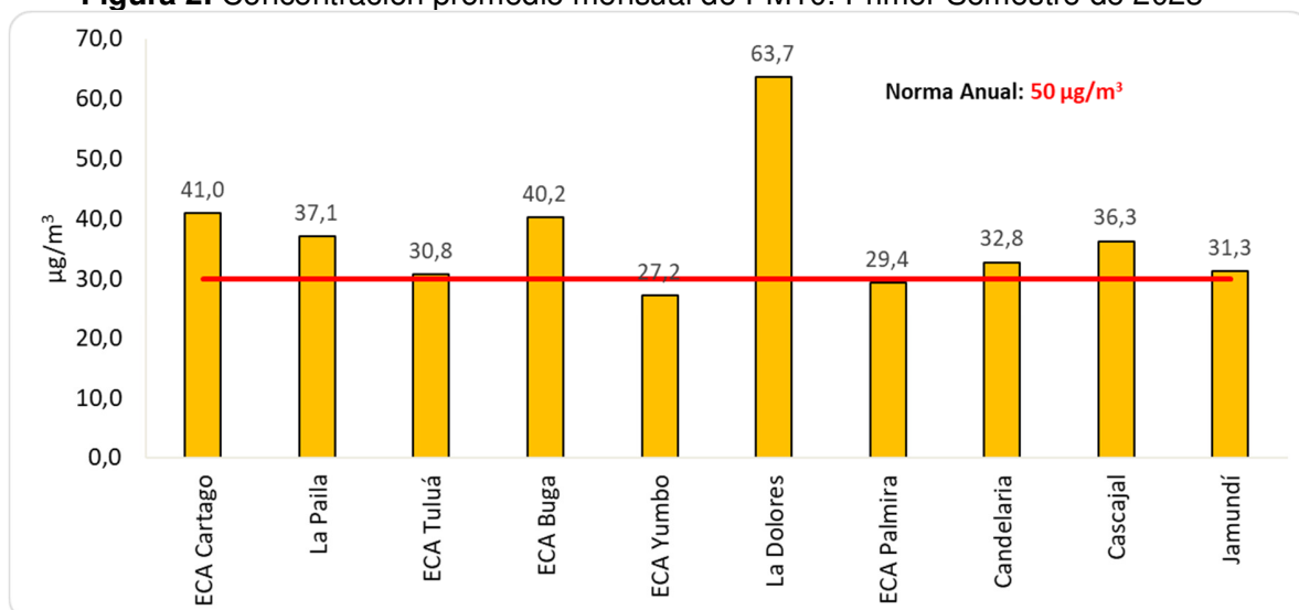
Figura 2. Concentración promedio mensual de PM10. Primer Semestre de 2023
