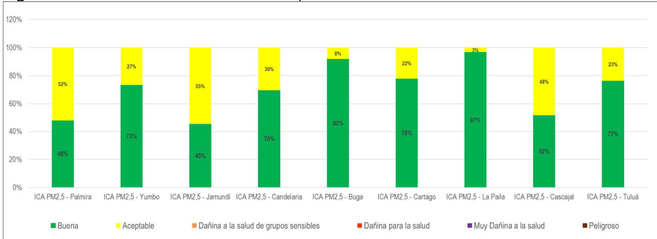
Figura 5. ICA de las concentraciones diarias promedio de PM2.5. Primer Semestre de 2023.
