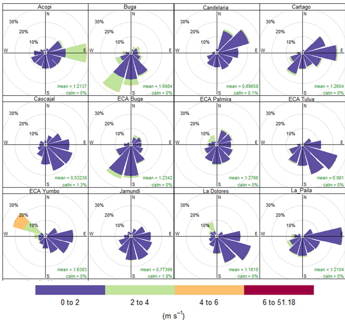
Figura 4. Rosa de los Vientos SVCA de la CVC. Primer Semestre de 2023
