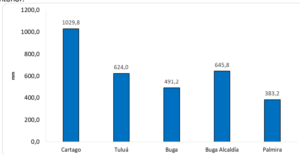
Figura 5. Precipitación acumulada en Primer Semestre de 2023.
