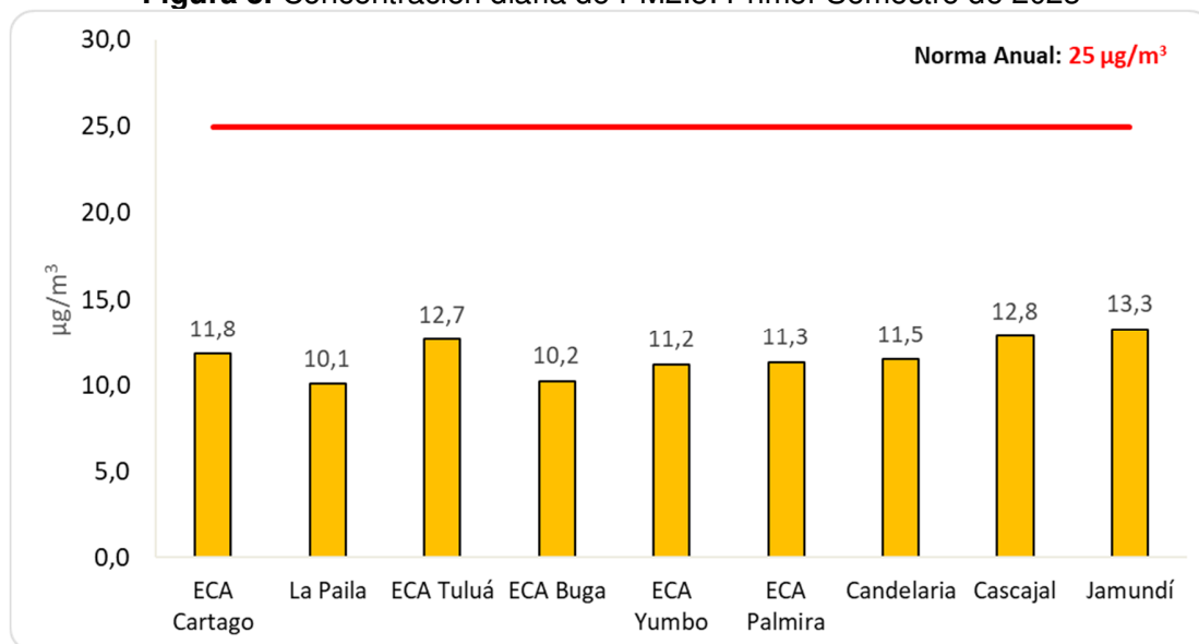
Figura 3. Concentración diaria de PM2.5. Primer Semestre de 2023
