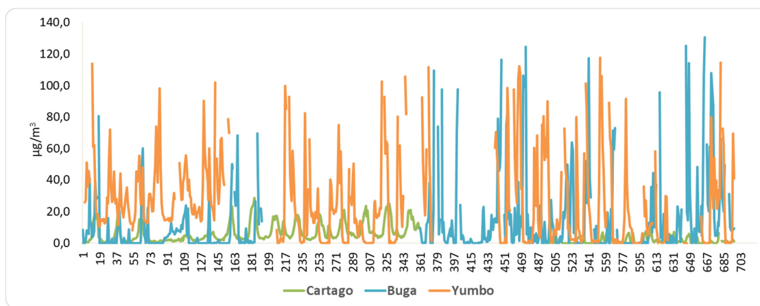
Figura 3. Concentración horaria de SO 2 . Febrero 2024
