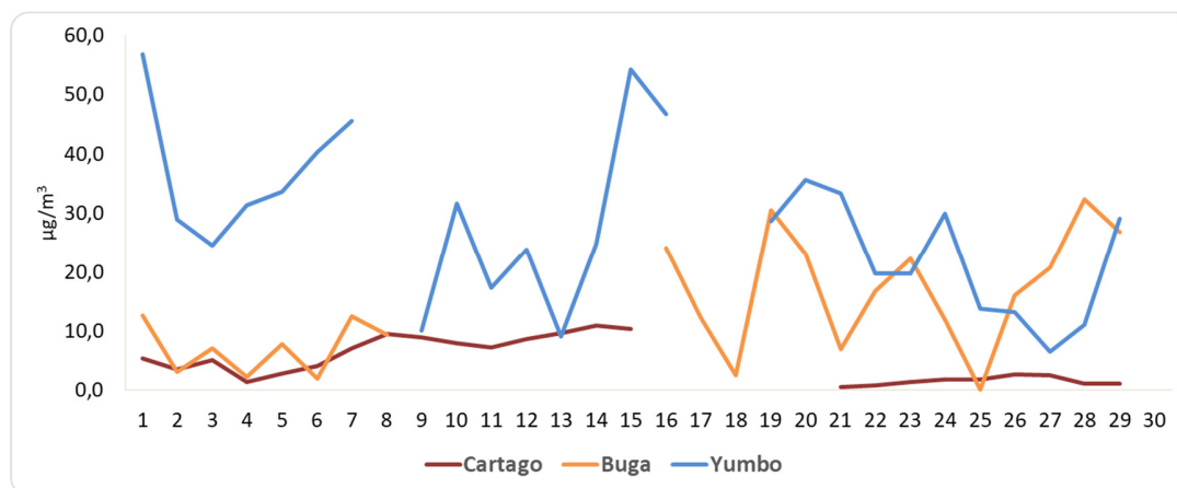
Figura 4. Concentración diaria de SO 2 . Febrero 2024
