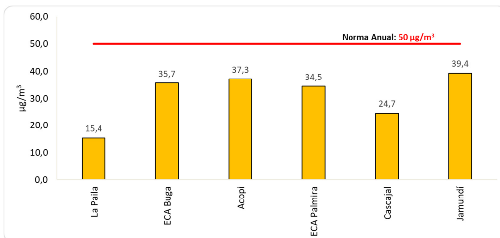
Figura 1. Concentración promedio mensual de PM10. Febrero 2024
