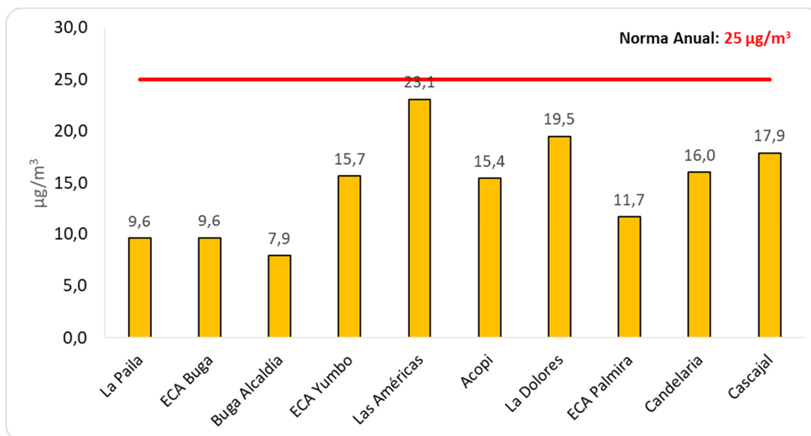
Figura 2. Concentración diaria de PM2.5. Febrero 2024
