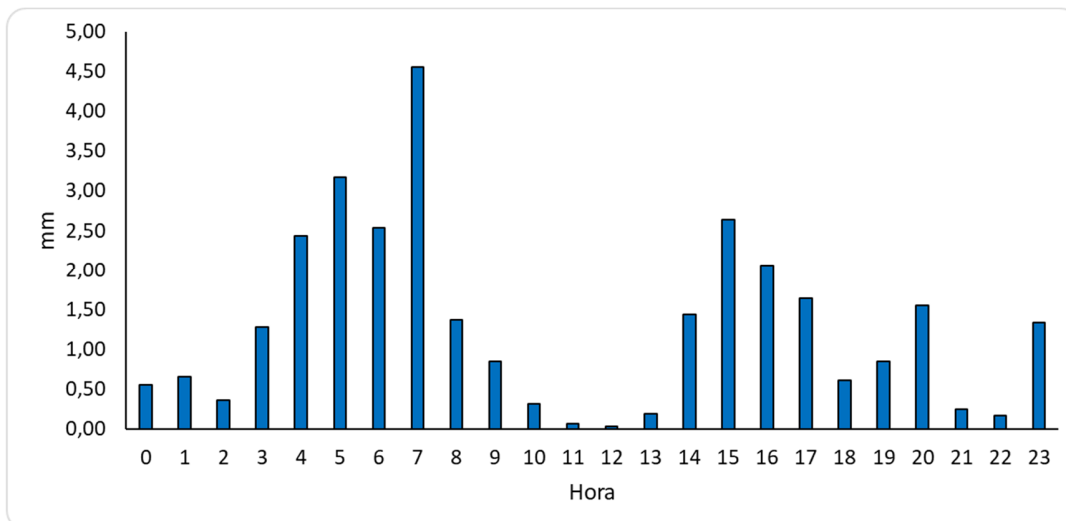
Figura 9. Precipitación acumulada horaria en Julio 2024
