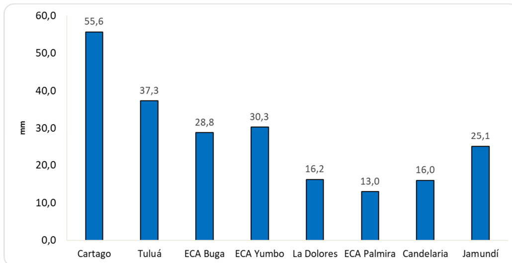
Figura 8. Precipitación acumulada en Julio 2024
