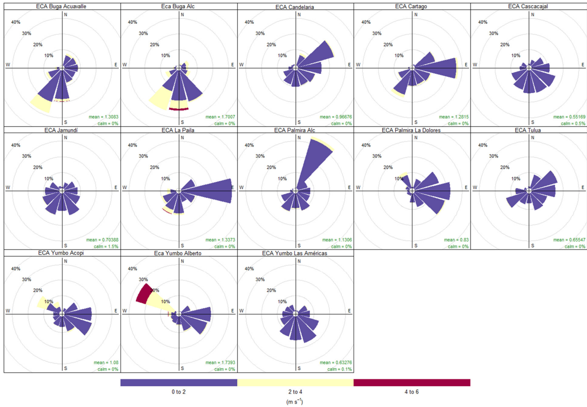
Figura 7. Rosa de los Vientos SVCA de la CVC. Julio 2024
