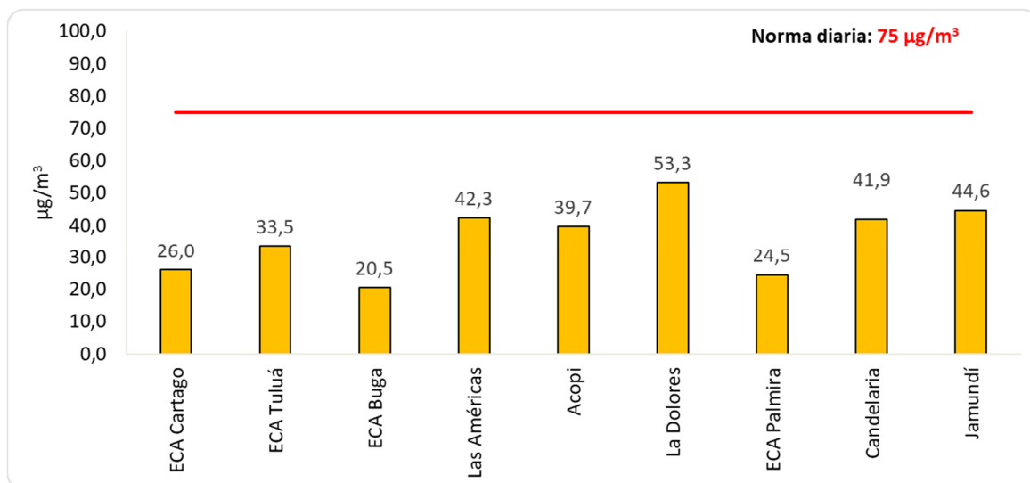
Figura 1. Concentración promedio mensual de PM10. Julio 2024
