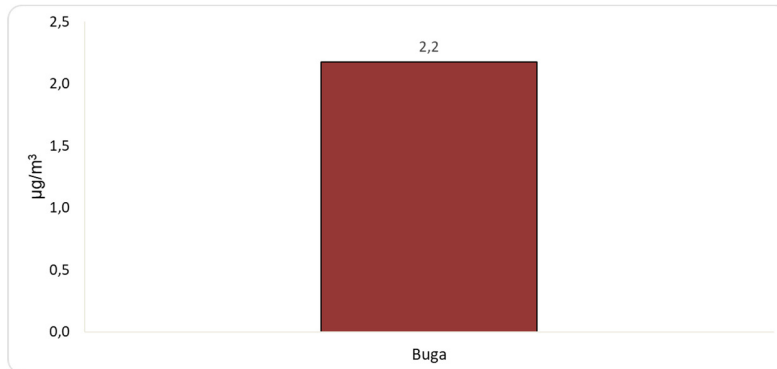
Figura 5. Promedio horario diario de NO 2 . Julio 2024
