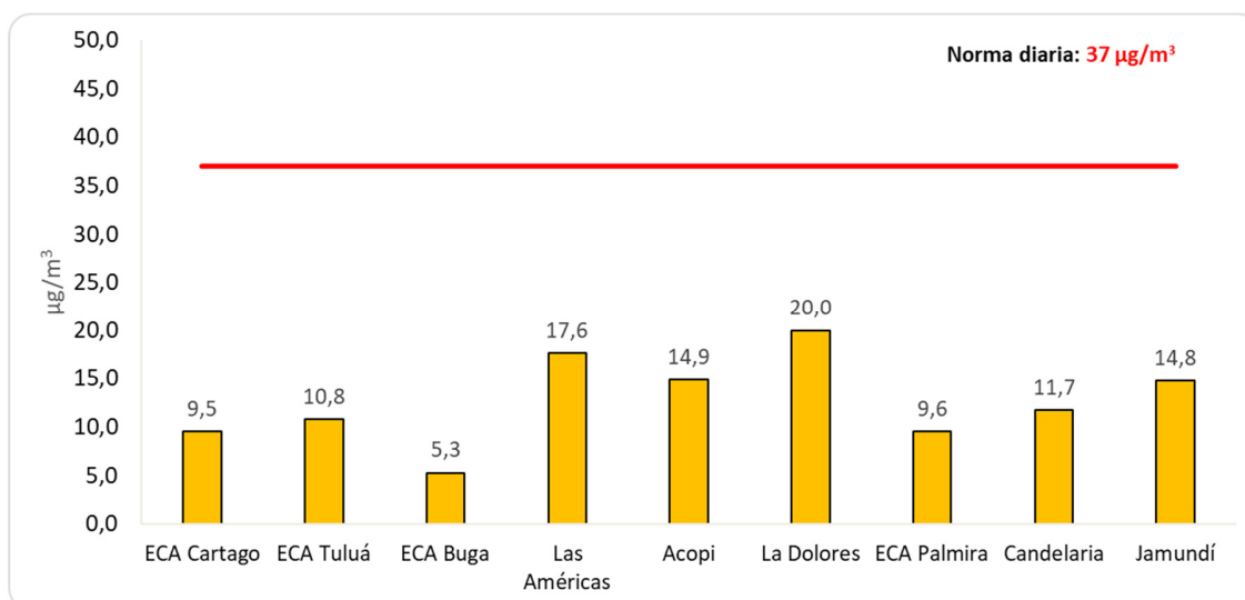
Figura 2. Concentración diaria de PM2.5. Julio 2024
