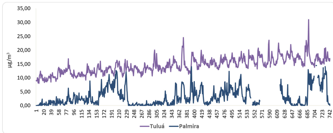
Figura 3. Concentración horaria de SO 2 . Julio 2024
