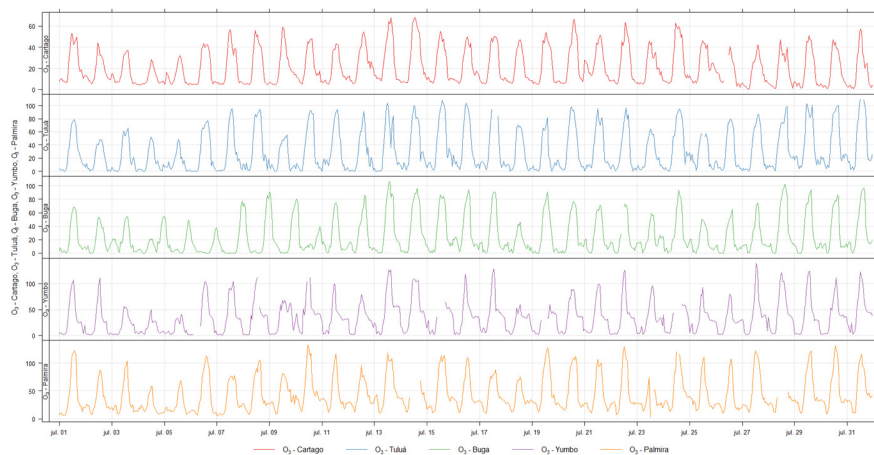
Figura 6. Promedio horario de O 3 . Julio 2024
