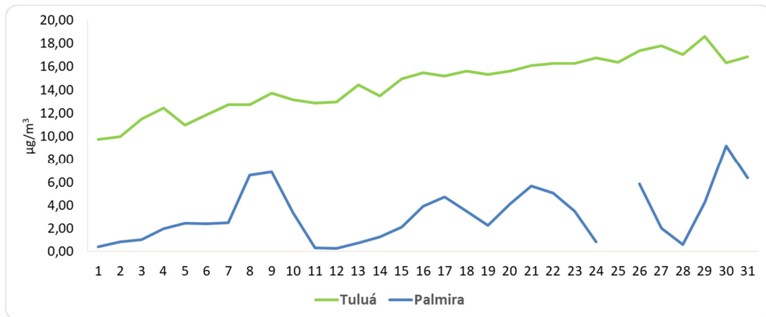
Figura 4. Concentración diaria de SO 2 . Julio 2024
