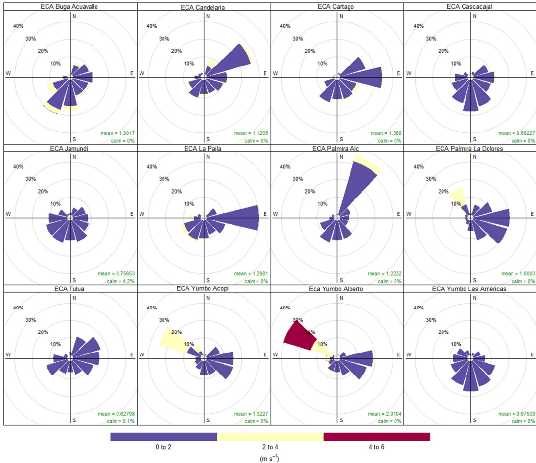
Figura 6. Rosa de los Vientos SVCA de la CVC. Agosto 2024
