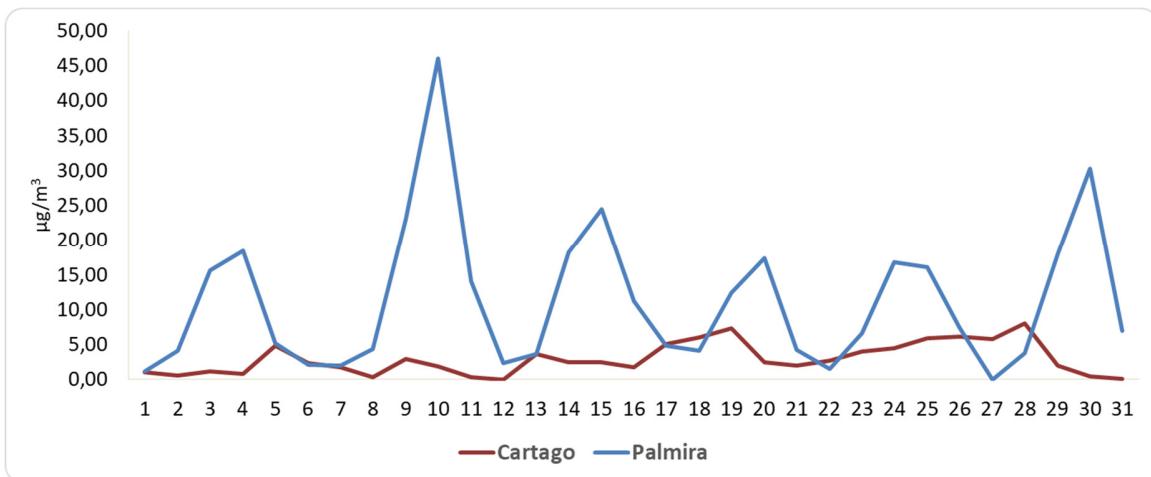
Figura 4. Concentración diaria de SO 2 . Agosto 2024
