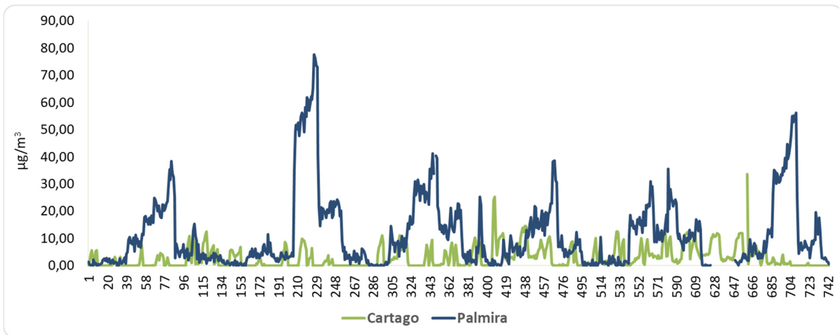
Figura 3. Concentración horaria de SO 2 . Agosto 2024
