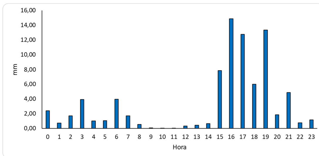
Figura 8. Precipitación acumulada horaria en Agosto 2024
