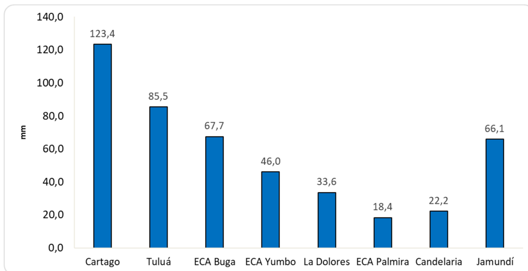
Figura 7. Precipitación acumulada en Agosto 2024
