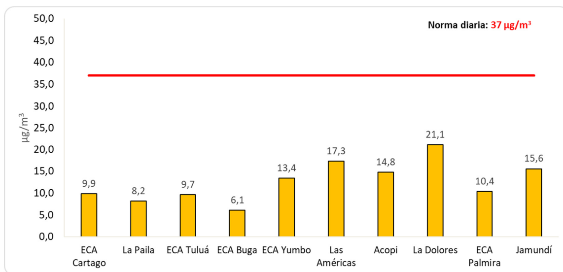
Figura 2. Concentración diaria de PM2.5. Agosto 2024
