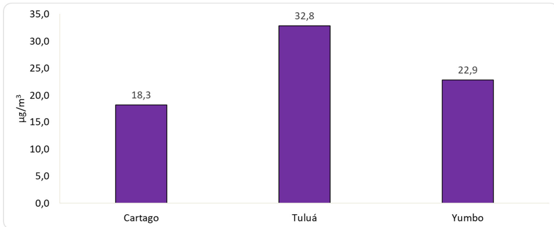
Figura 5. Promedio horario de O 3 . Agosto 2024
