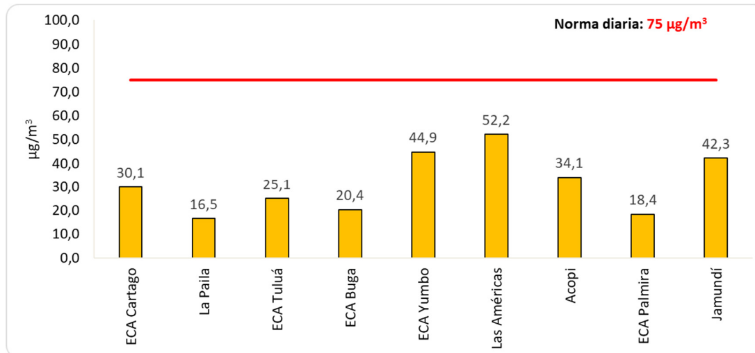
Figura 1. Concentración promedio mensual de PM10. Agosto 2024
