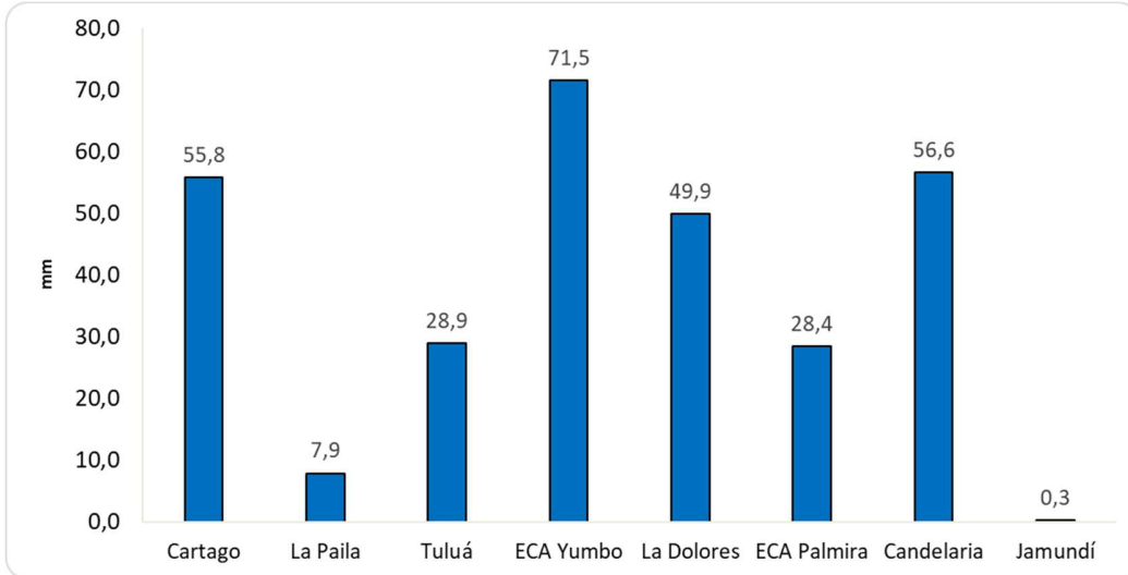
Figura 8. Precipitación acumulada en Septiembre 2024
