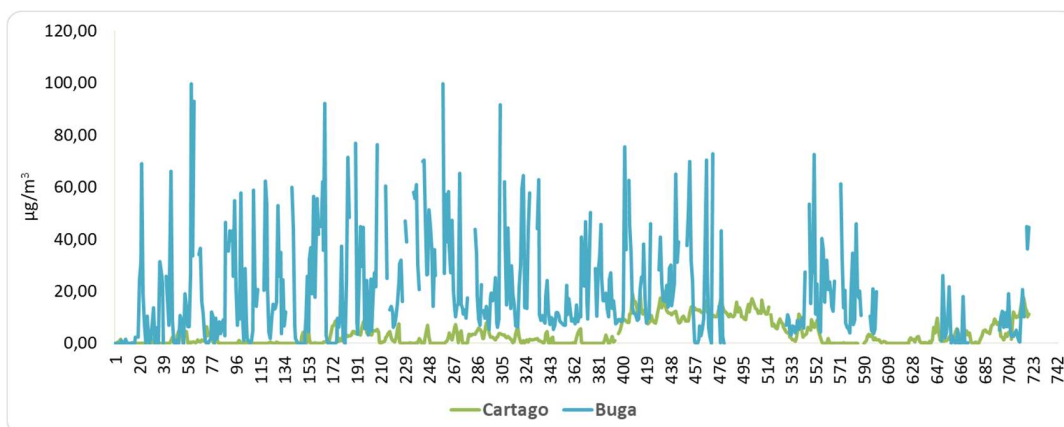
Figura 3. Concentración horaria promedio de SO 2 . Septiembre 2024
