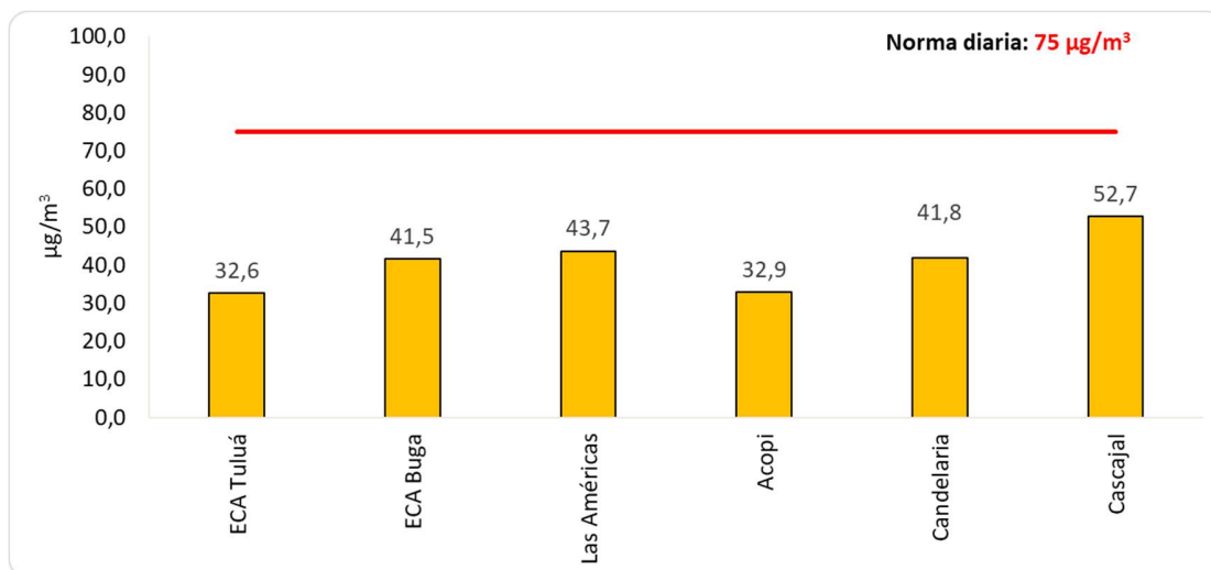
Figura 1. Concentración promedio mensual de PM10. Septiembre 2024
