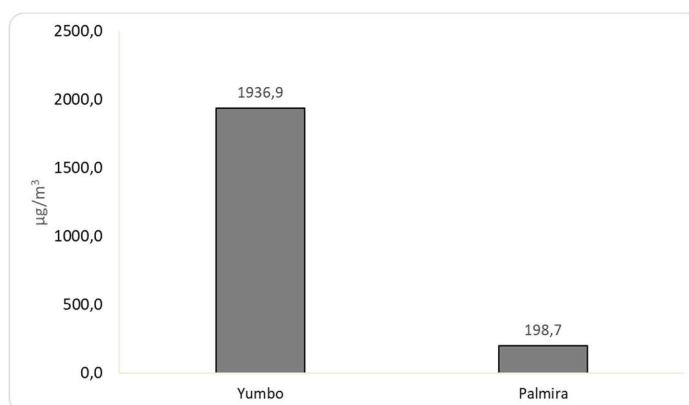
Figura 4. Promedio octo horario diario de O 3 . Tercer Trimestre 2024
