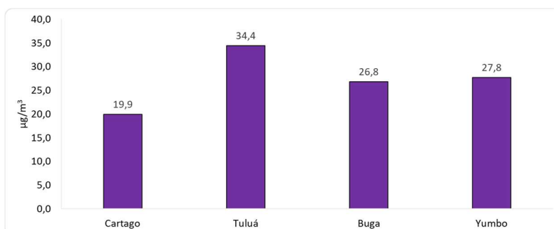
Figura 3. Promedio octo horario diario de O 3 . Tercer Trimestre 2024
