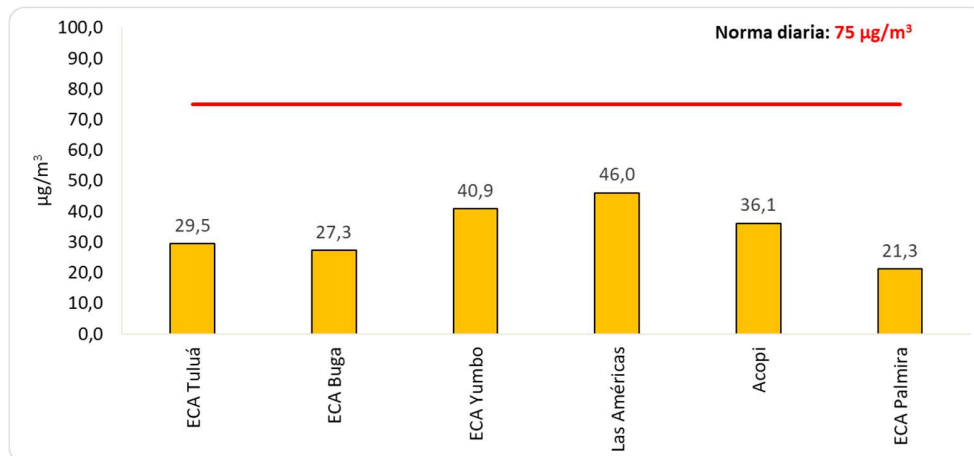
Figura 1. Concentración diaria promedio de PM10. Tercer Trimestre 2024
