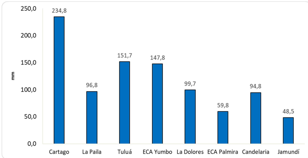
Figura 6. Precipitación acumulada en Tercer Trimestre 2024
