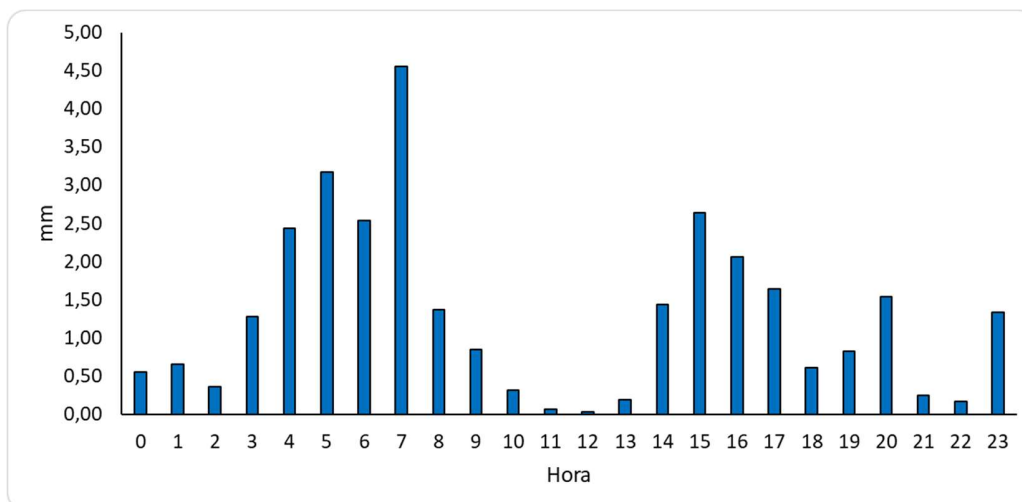
Figura 7. Precipitación acumulada horaria. Tercer Trimestre 2024
