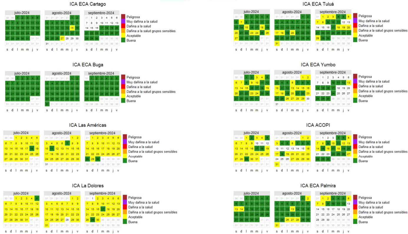
Figura 9. ICA de las concentraciones diarias promedio de PM2.5. Tercer Trimestre 2024
