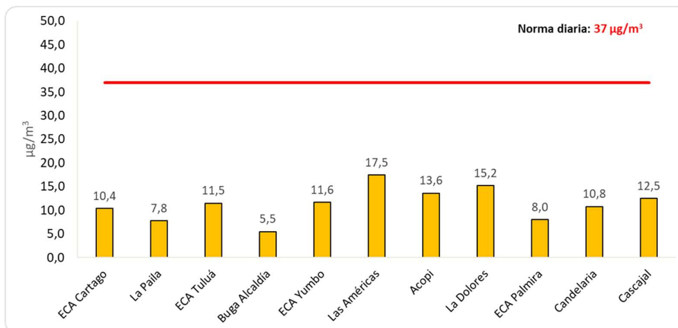
Figura 2. Concentración diaria promedio de PM2.5. Tercer Trimestre 2024
