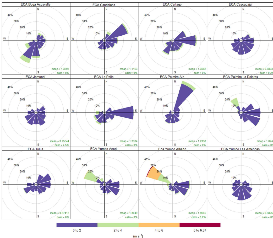
Figura 5. Rosa de los Vientos SVCA de la CVC. Tercer Trimestre 2024
