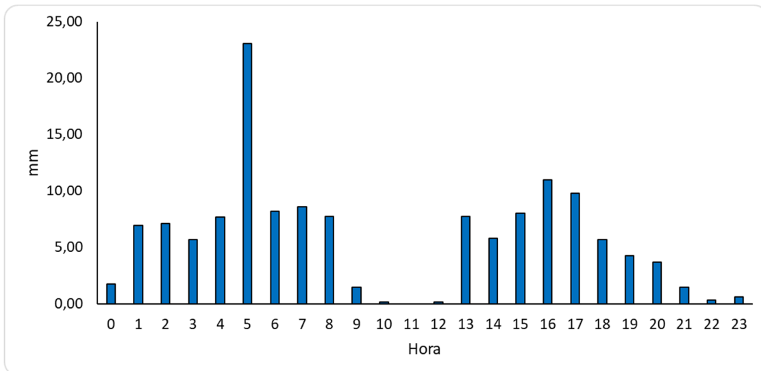
Figura 8. Precipitación acumulada horaria en Octubre 2024
