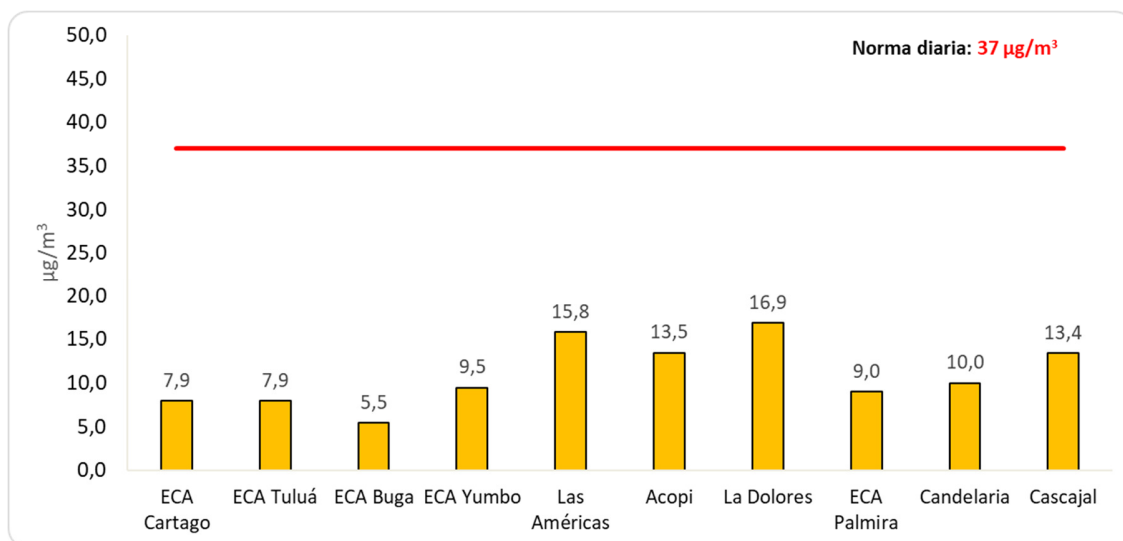
Figura 2. Concentración diaria de PM2.5. Octubre 2024
