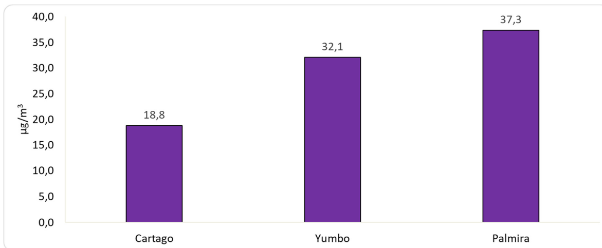
Figura 5. Promedio horario de O 3 . Octubre 2024
