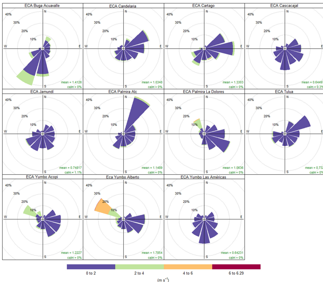
Figura 6. Rosa de los Vientos SVCA de la CVC. Octubre 2024
