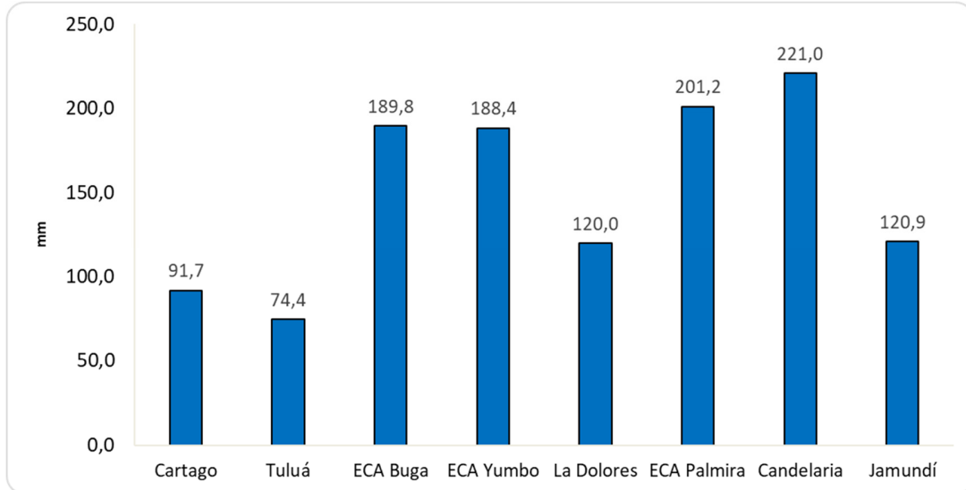
Figura 7. Precipitación acumulada en octubre 2024
