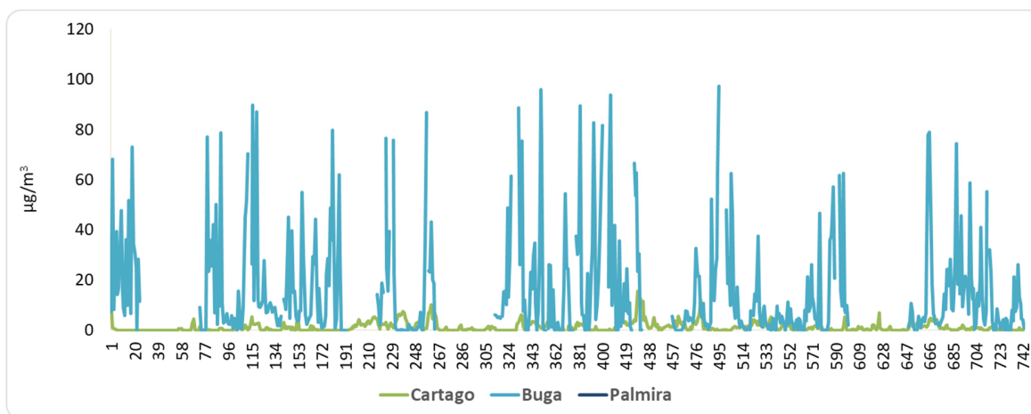
Figura 3. Concentración horaria promedio de SO 2 . Octubre 2024
