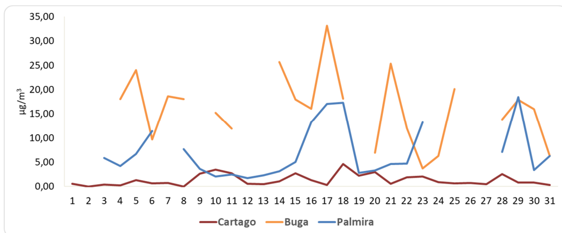
Figura 4. Concentración diaria promedio de SO 2 . Octubre 2024
