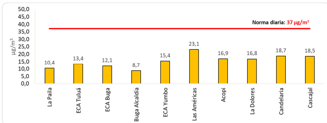
Figura 2. Concentración diaria de PM2.5. Enero 2024
