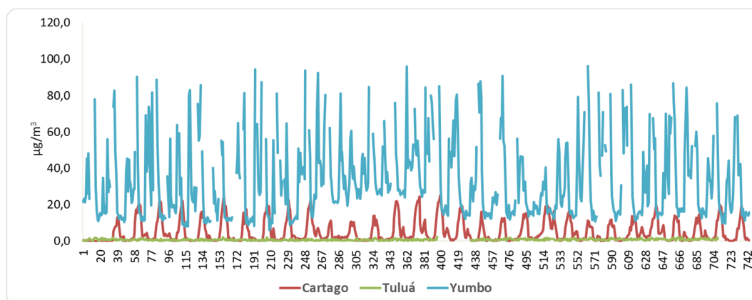
Figura 3. Concentración horaria de SO 2 . Enero 2024
