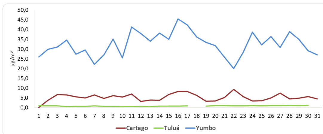
Figura 4. Concentración diaria de SO 2 . Enero 2024
