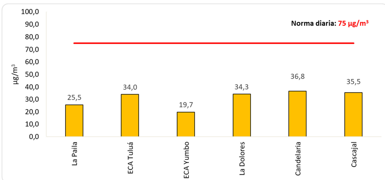
Figura 1. Concentración promedio mensual de PM10. Enero 2024
