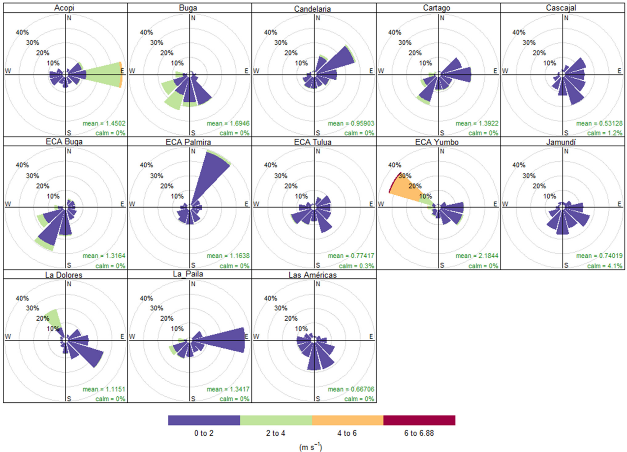
Figura 6. Rosa de los Vientos SVCA de la CVC. Enero 2024
