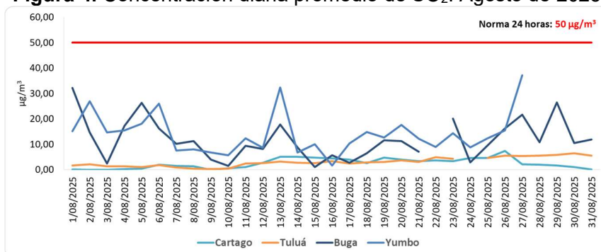
Figura 4. Concentración diaria promedio de SO 2 . Agosto de 2025
