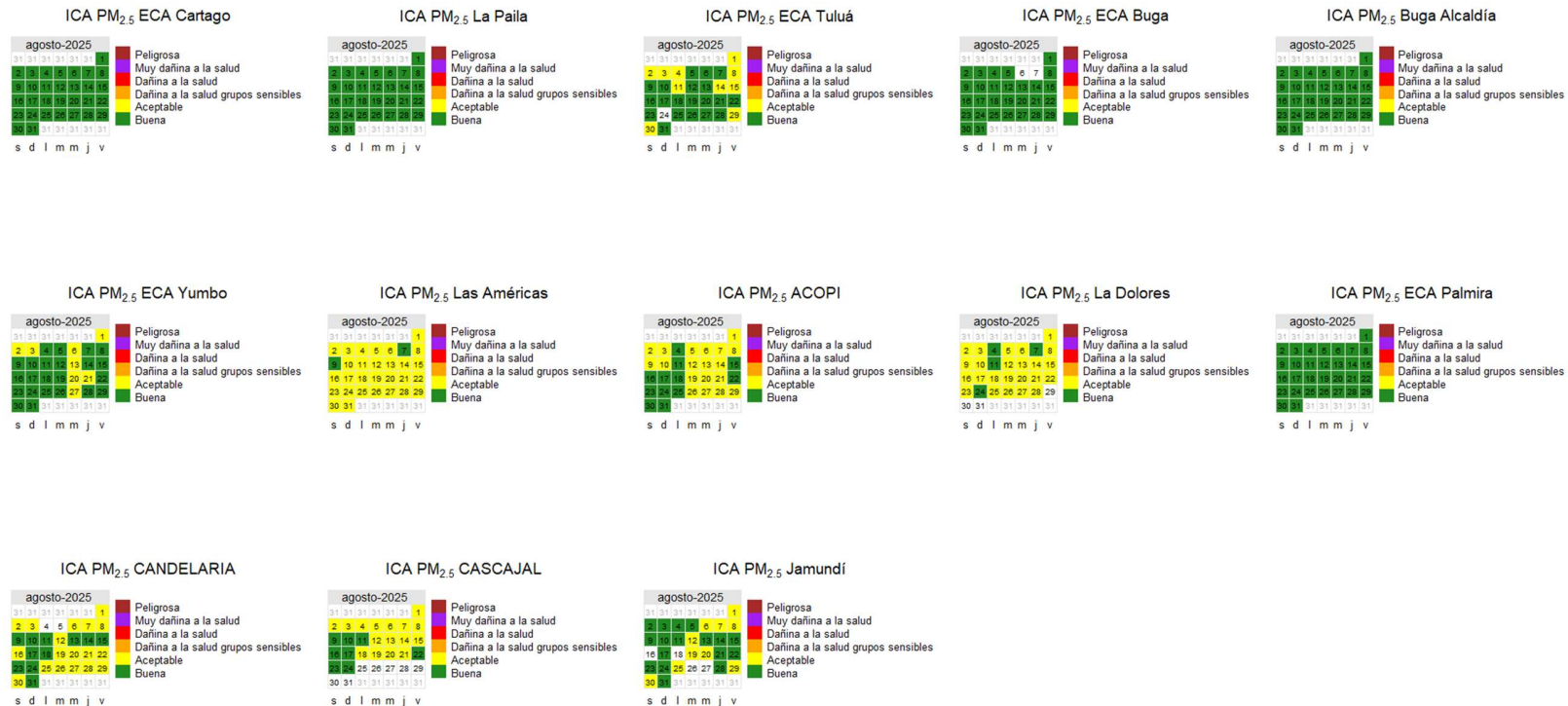
Figura 19. ICA de las concentraciones diarias promedio de PM2.5. Agosto de 2025
