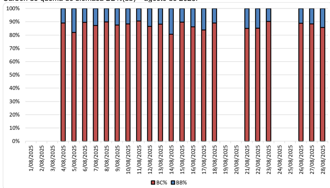
Figura 12. Serie temporal porcentaje de quema Black Carbón de combustibles fósiles BC%(ff) vs. Black Carbón de quema de biomasa BB%(bb) – agosto de 2025.
