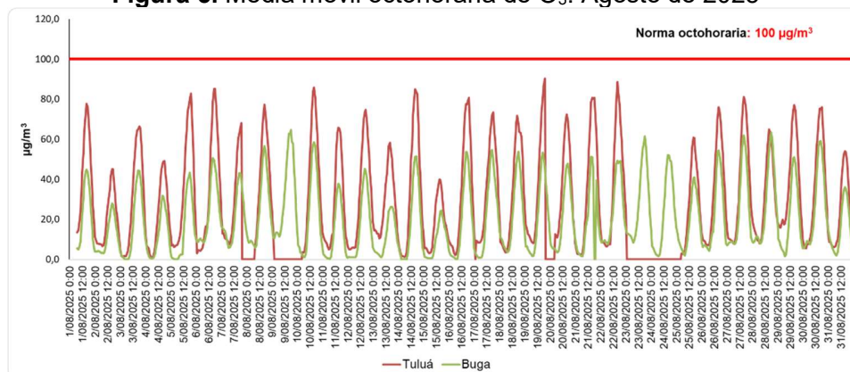
Figura 5. Media móvil octohoraria de O 3 . Agosto de 2025
