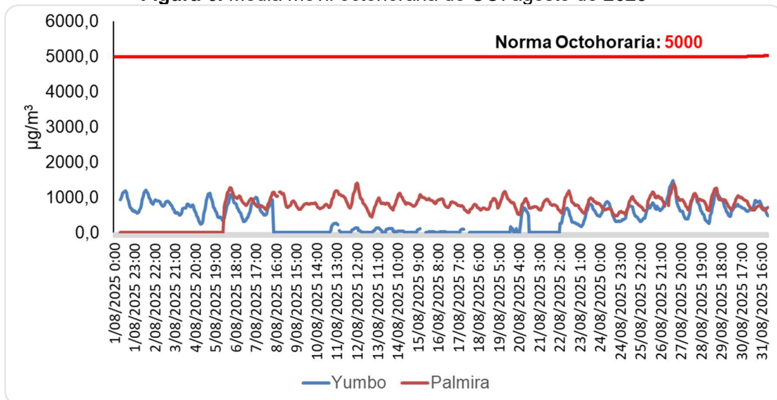
Figura 6. Media móvil octohoraria de CO. agosto de 2025
