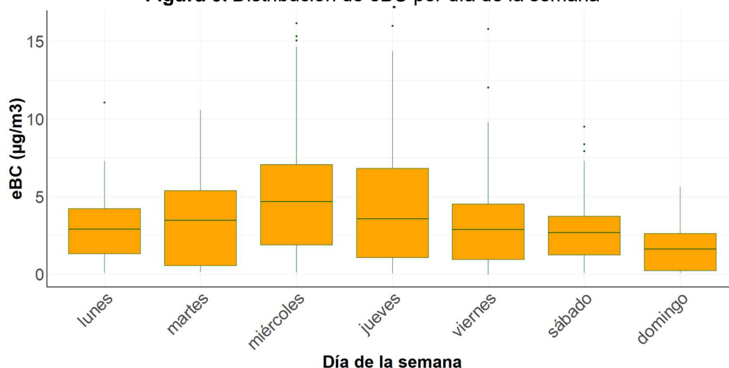
Figura 9. Distribución de eBC por día de la semana
