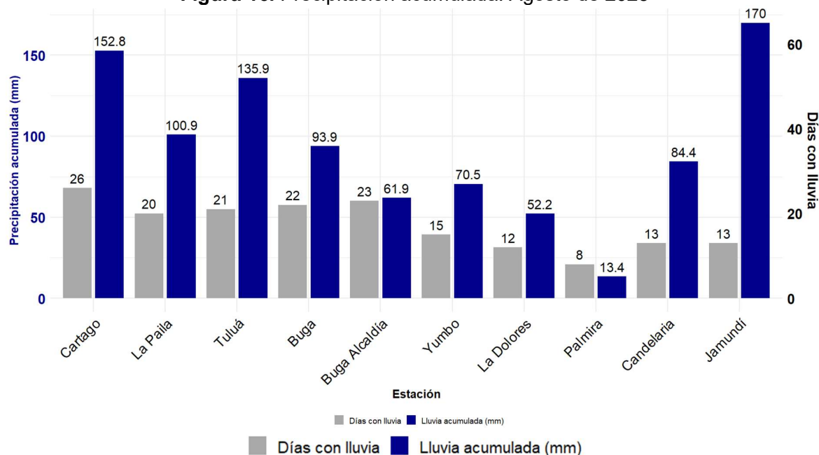
Figura 16. Precipitación acumulada. Agosto de 2025
