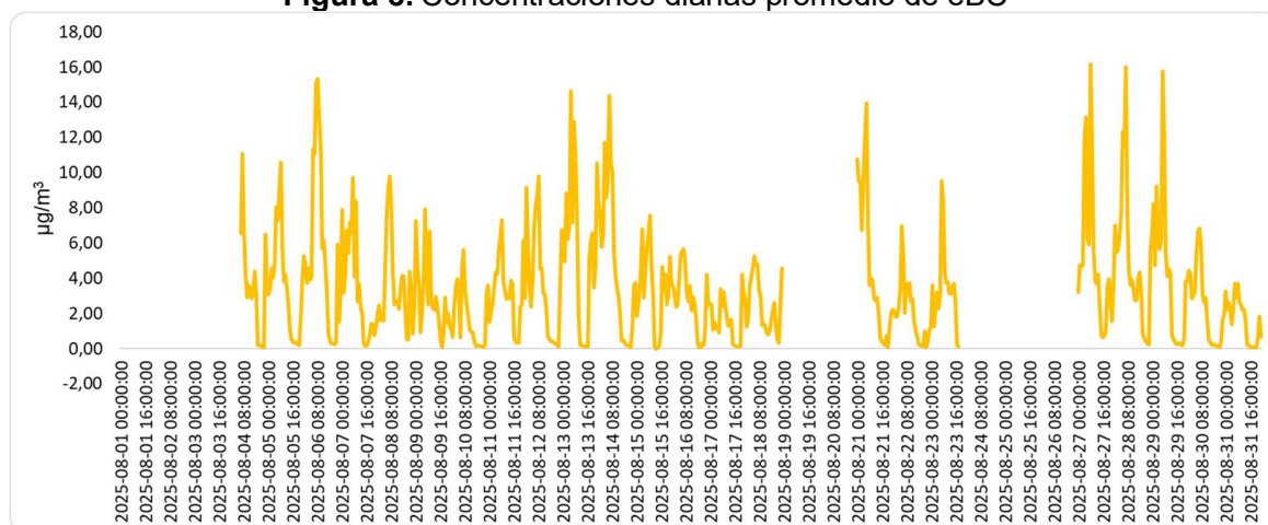
Figura 8. Concentraciones diarias promedio de eBC
