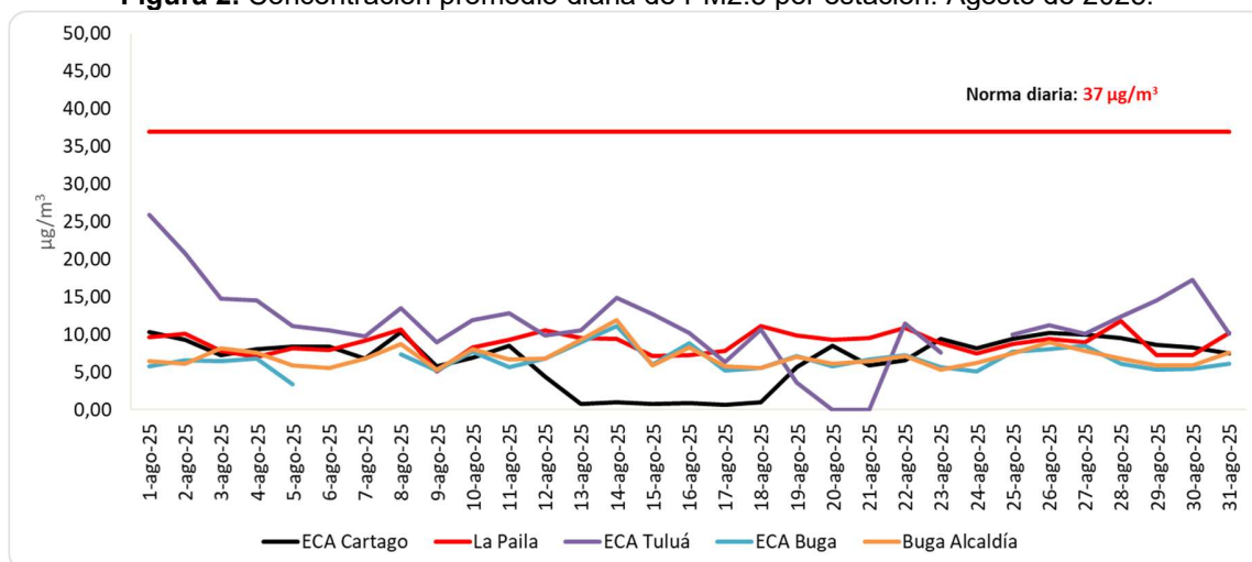
Figura 2. Concentración promedio diaria de PM2.5 por estación. Agosto de 2025.
