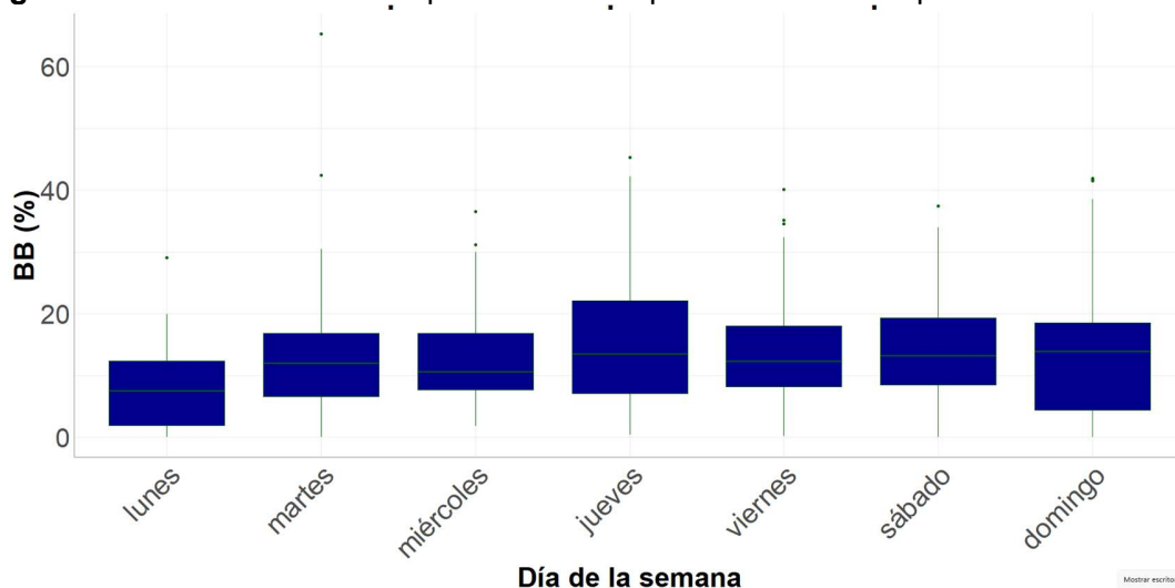
Figura 11. Distribución de eBC proveniente de quema de biomasa por día de la semana
