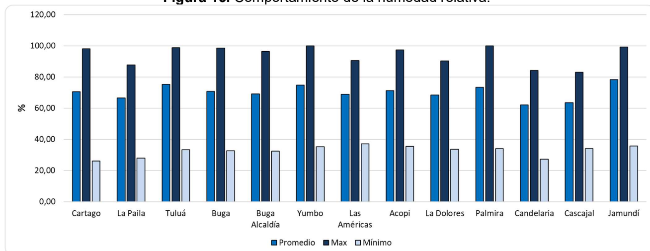
Figura 15. Comportamiento de la humedad relativa.
