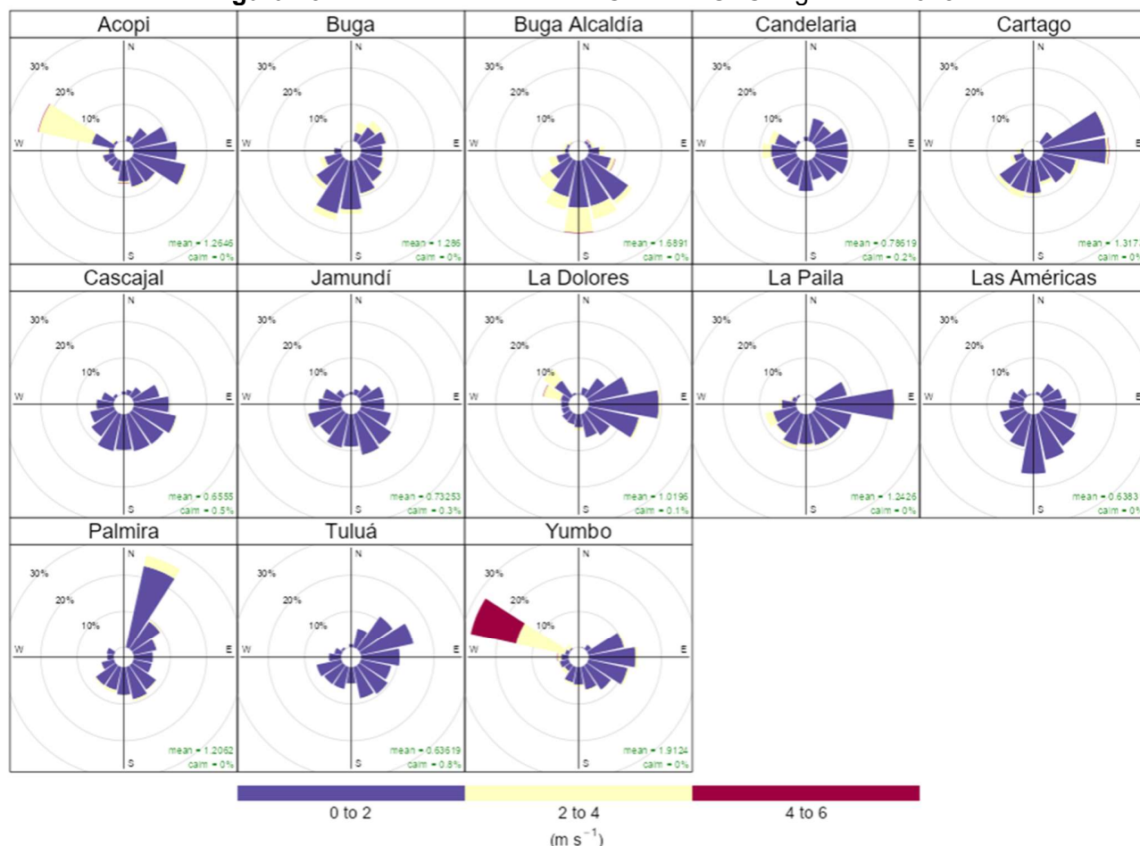
Figura 13. Rosa de los Vientos SVCA de la CVC. Agosto de 2025
