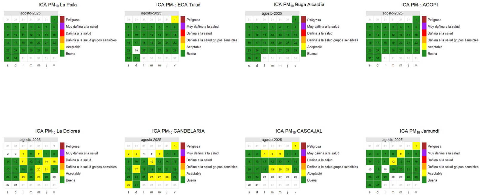
Figura 18. ICA de PM 10 . Agosto de 2025
