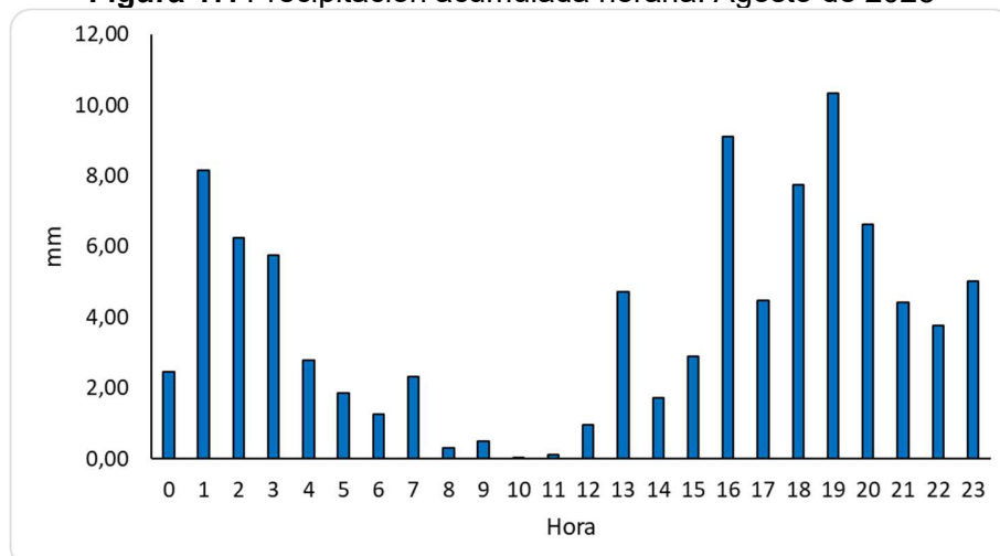
Figura 17. Precipitación acumulada horaria. Agosto de 2025
