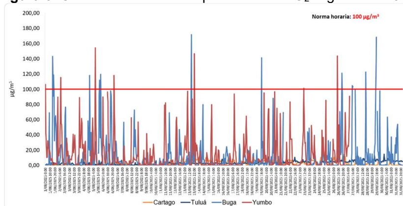
Figura 3. Concentración horaria promedio de SO 2 . Agosto de 2025
