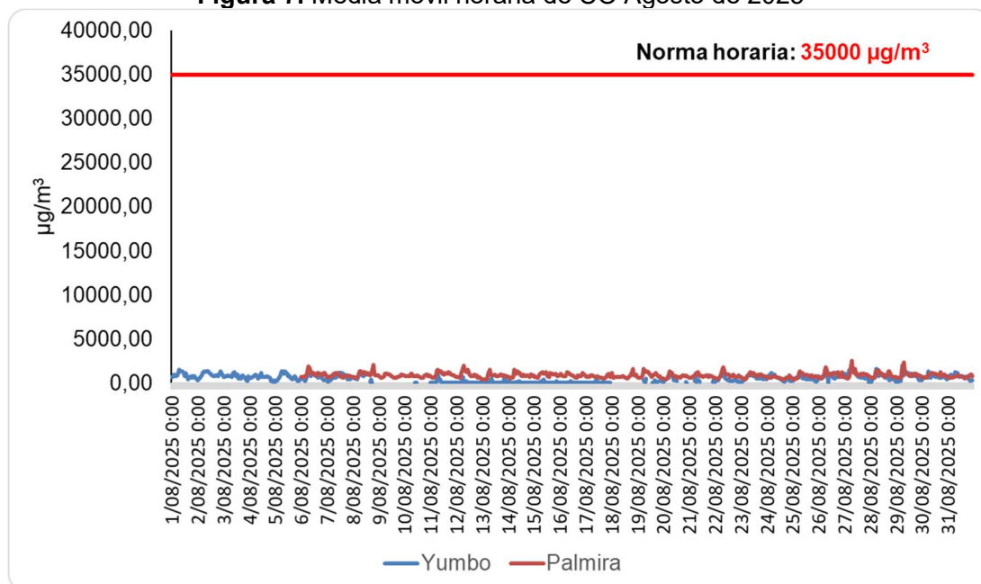
Figura 7. Media móvil horaria de CO Agosto de 2025
