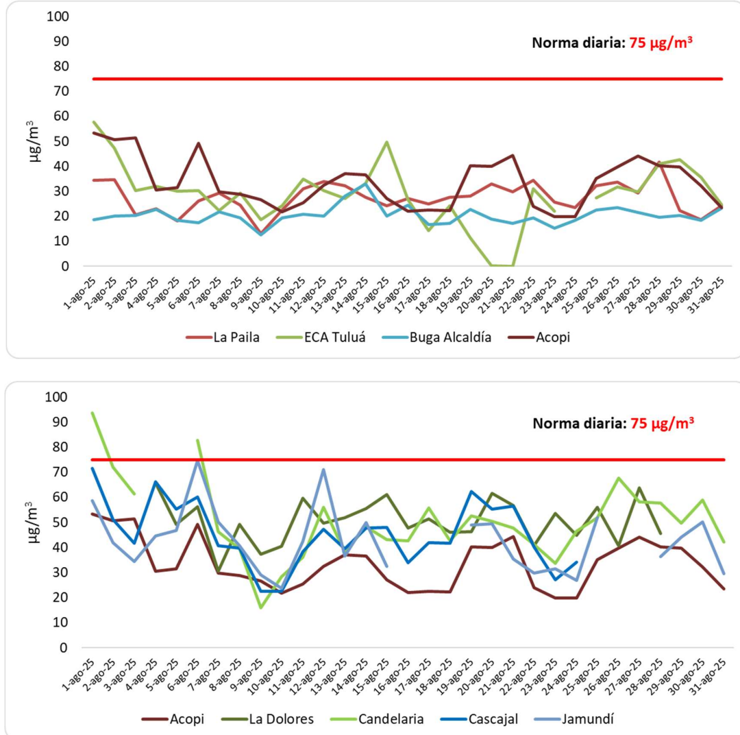
Figura 1. Concentración promedio diaria de PM10 por estación. Agosto de 2025
