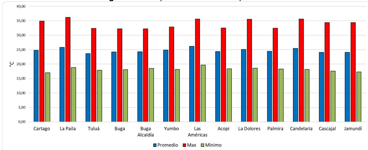
Figura 14. Comportamiento de la temperatura.
