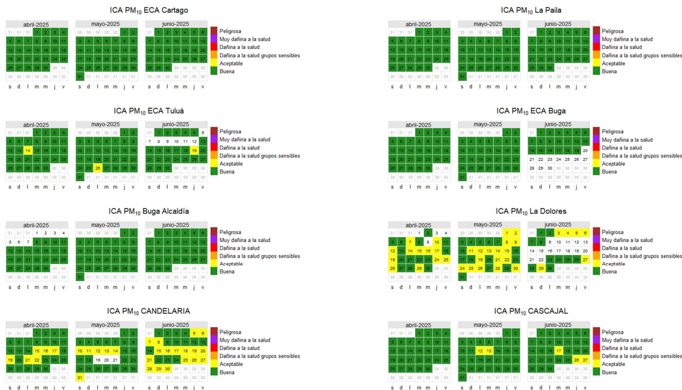
Figura 11. ICA de PM10. Segundo trimestre de 2025
