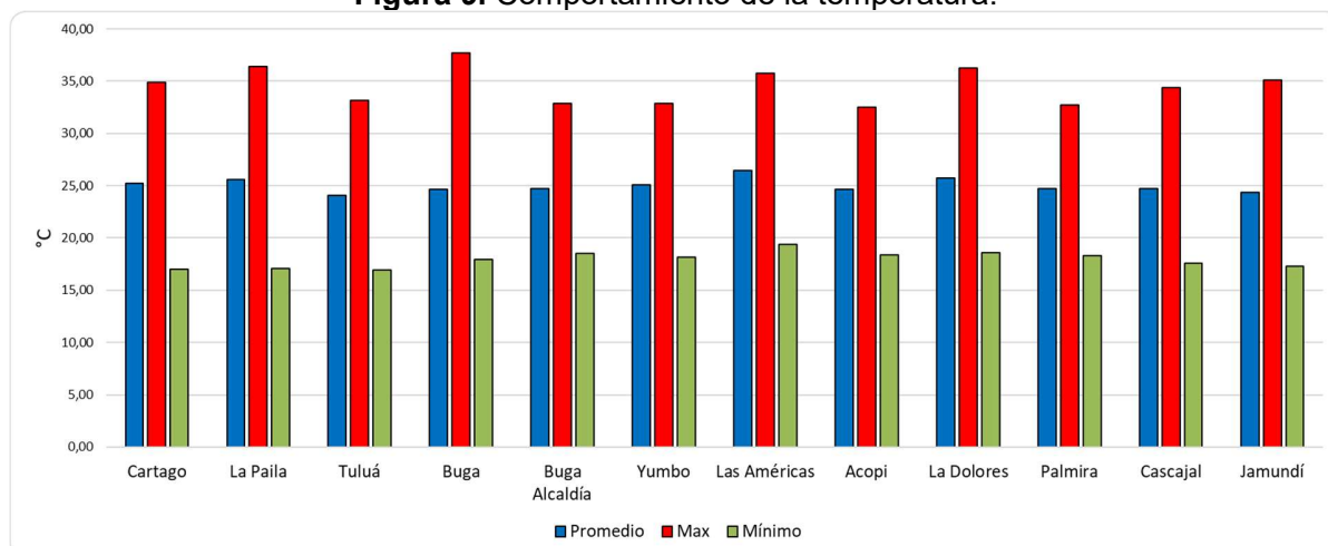
Figura 9. Comportamiento de la temperatura.
