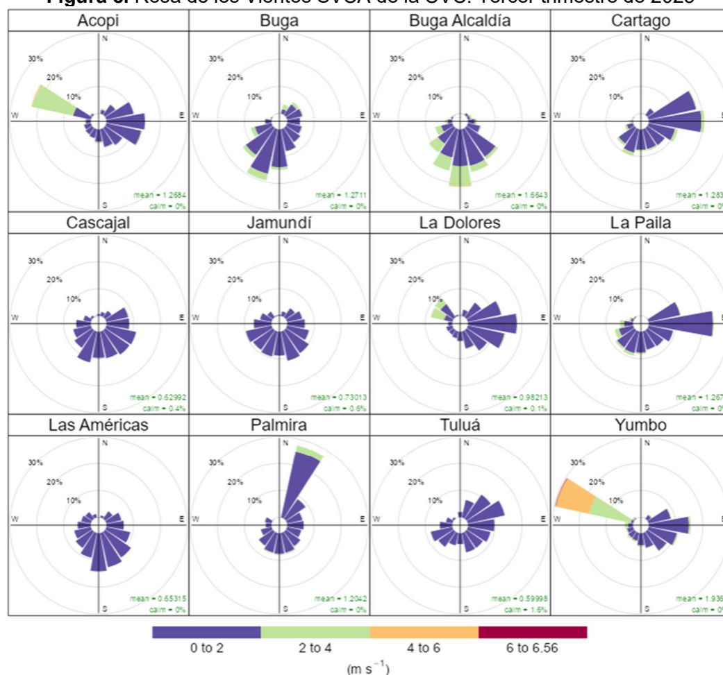
Figura 8. Rosa de los Vientos SVCA de la CVC. Tercer trimestre de 2025
