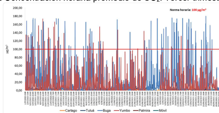
Figura 3. Concentración horaria promedio de SO 2 . Tercer trimestre de 2025
