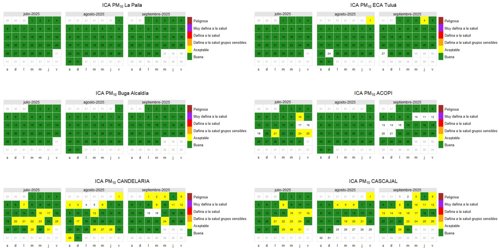
Figura 13. ICA de PM 10 . Tercer trimestre de 2025
