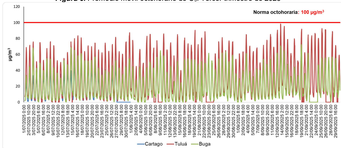
Figura 5. Promedio móvil octohorario de O 3 . Tercer trimestre de 2025
