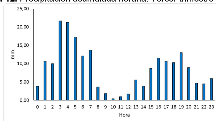
Figura 12. Precipitación acumulada horaria. Tercer trimestre de 2025
