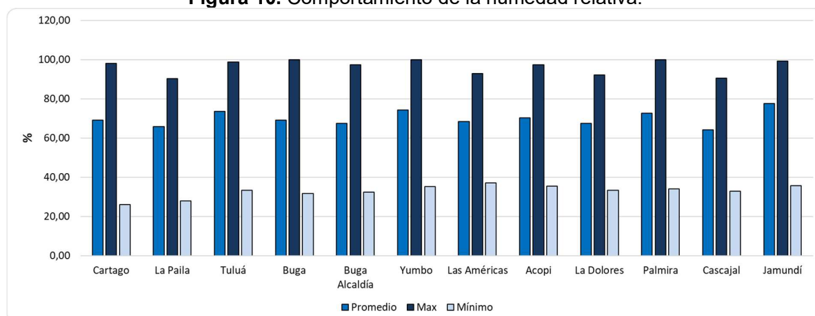
Figura 10. Comportamiento de la humedad relativa.
