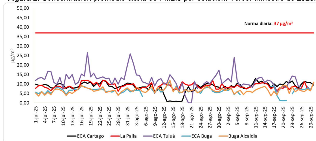
Figura 2. Concentración promedio diaria de PM2.5 por estación. Tercer trimestre de 2025.
