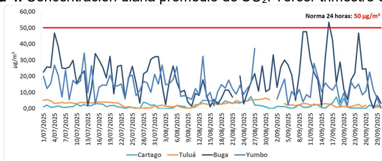
Figura 4. Concentración diaria promedio de SO 2 . Tercer trimestre de 2025
