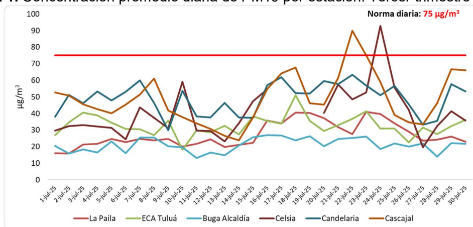
Figura 1. Concentración promedio diaria de PM10 por estación. Tercer trimestre de 2025
