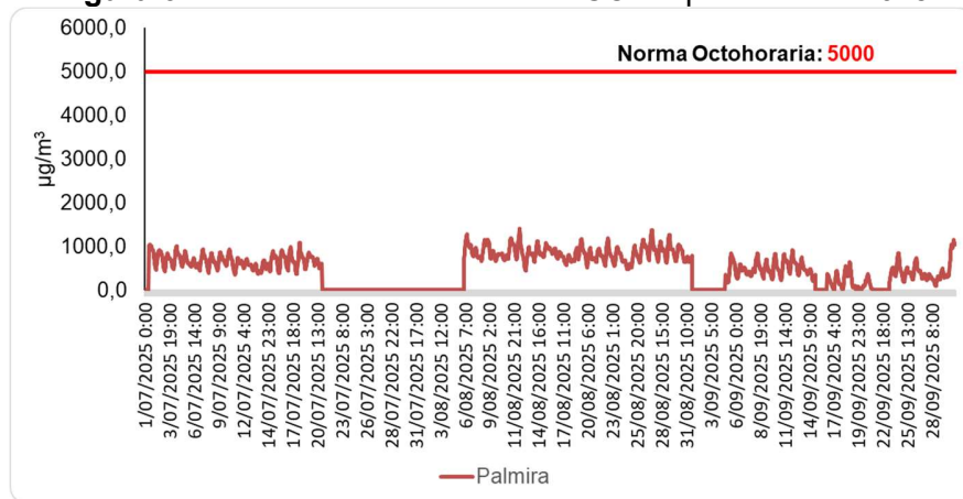
Figura 6. Media móvil octohoraria de CO. Septiembre de 2025
