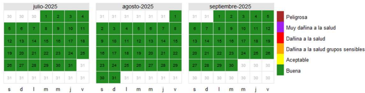
ICA PM 2.5 Buga Alcaldía
