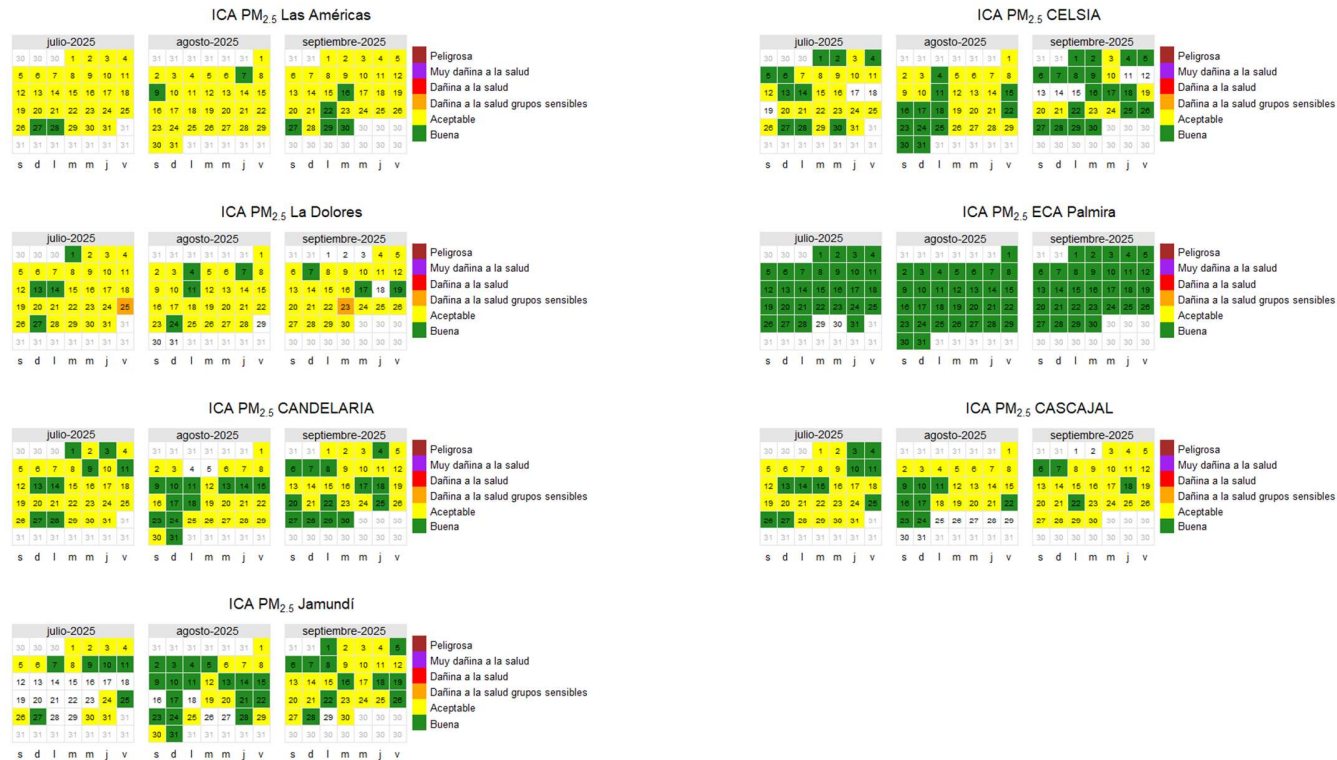
Figura 14. ICA de las concentraciones diarias promedio de PM2.5. Tercer trimestre de 2025
