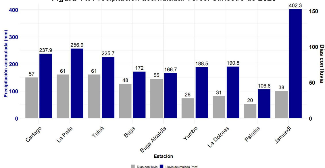
Figura 11. Precipitación acumulada. Tercer trimestre de 2025
