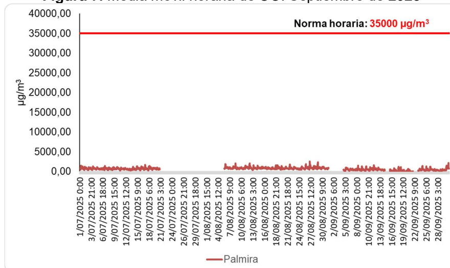
Figura 7. Media móvil horaria de CO. Septiembre de 2025
