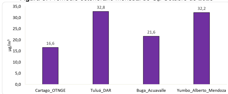
Figura 5. Promedio octohorario mensual de O 3 . Octubre de 2025
