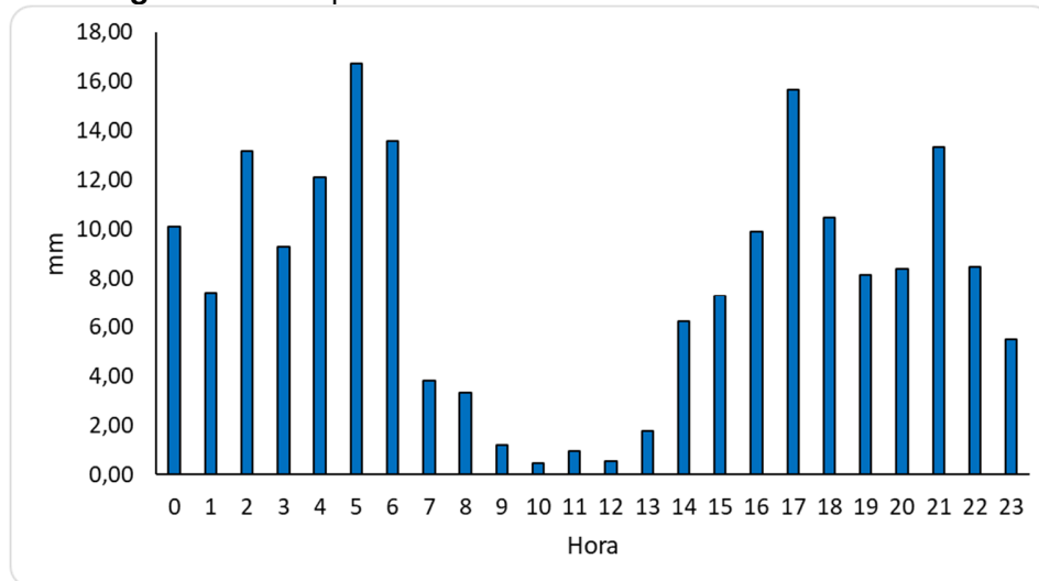
Figura 18. Precipitación acumulada horaria. Octubre de 2025
