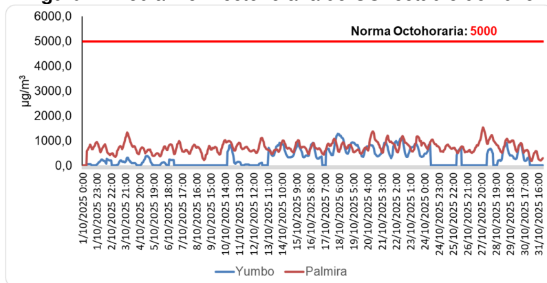
Figura 7. Media móvil octohoraria de CO. octubre de 2025
