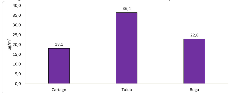
Figura 5. Promedio octohorario mensual de O 3 . Septiembre de 2025
