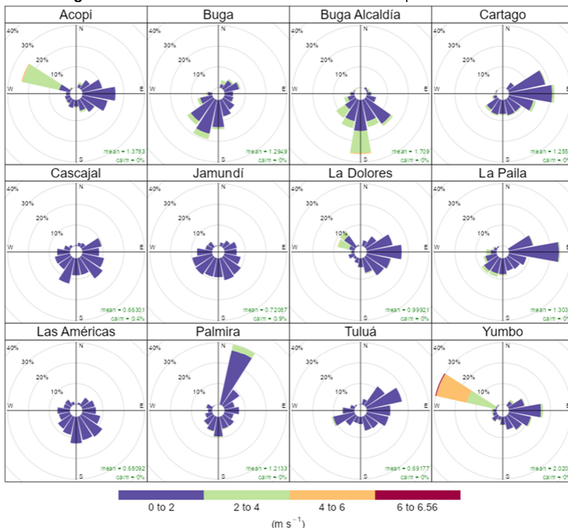
Figura 14. Rosa de los Vientos SVCA de la CVC. Septiembre de 2025
