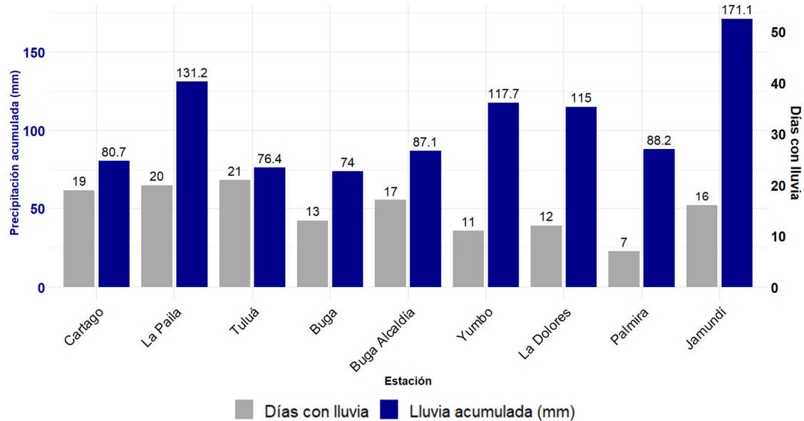
Figura 17. Precipitación acumulada. Septiembre de 2025
