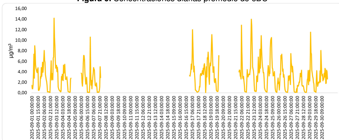
Figura 9. Concentraciones diarias promedio de eBC
