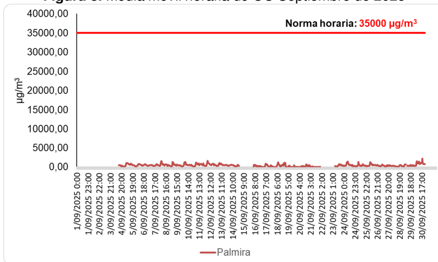
Figura 8. Media móvil horaria de CO Septiembre de 2025
