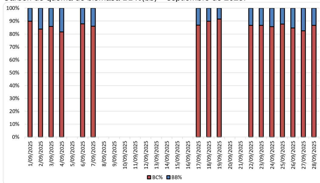
Figura 13. Serie temporal porcentaje de quema Black Carbón de combustibles fósiles BC%(ff) vs. Black Carbón de quema de biomasa BB%(bb) – septiembre de 2025.
