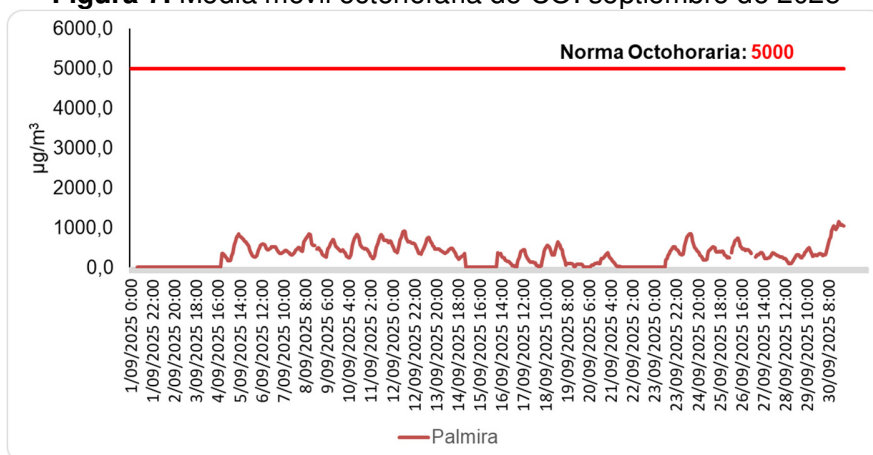
Figura 7. Media móvil octohoraria de CO. septiembre de 2025
