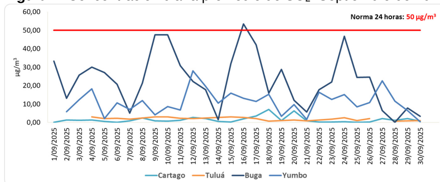
Figura 4. Concentración diaria promedio de SO 2 . Septiembre de 2025
