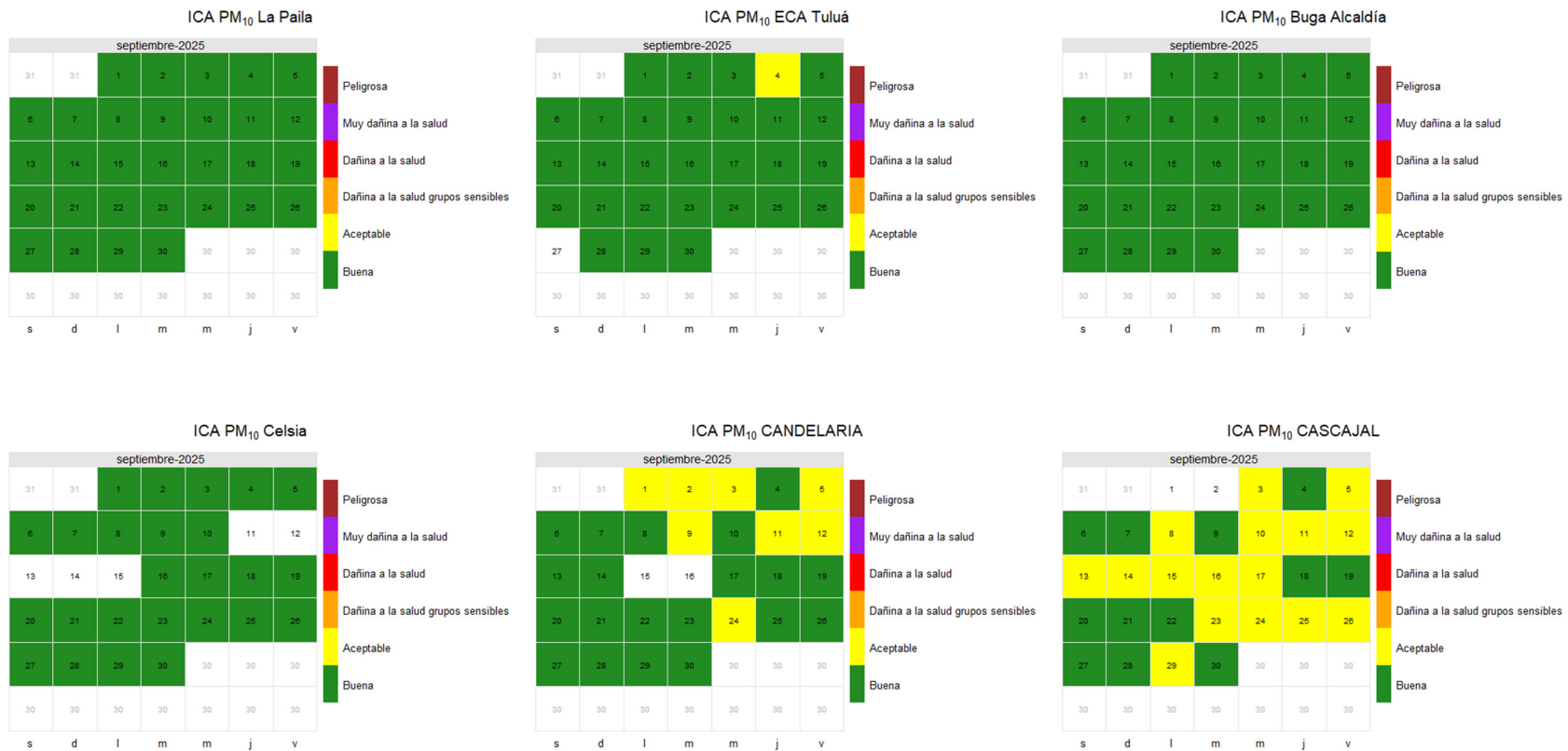
Figura 19. ICA de PM10. Septiembre de 2025
