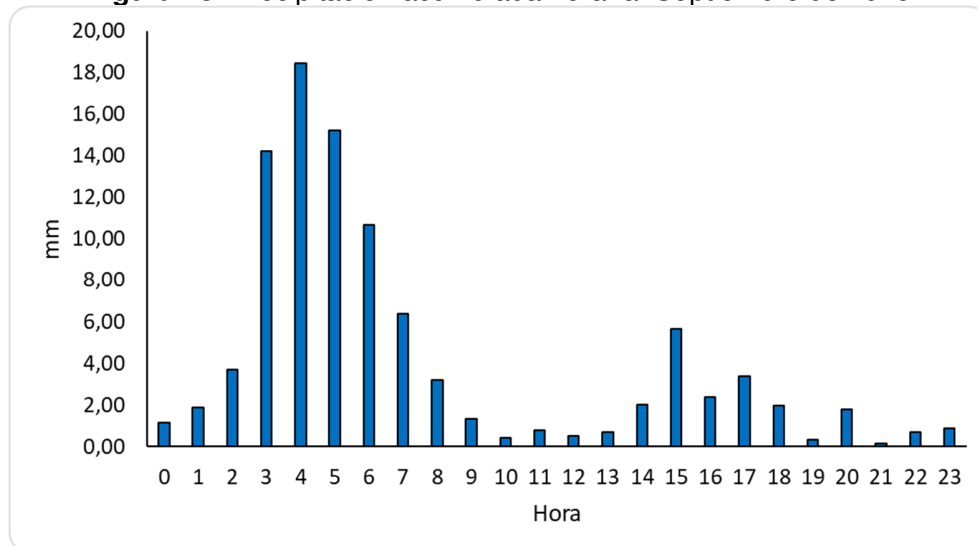
Figura 18. Precipitación acumulada horaria. Septiembre de 2025
