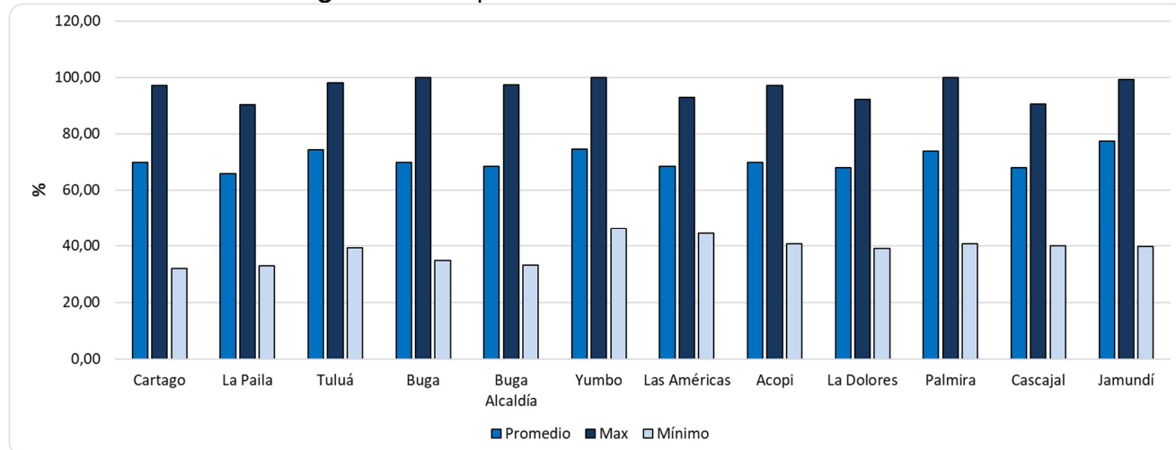
Figura 16. Comportamiento de la humedad relativa.
