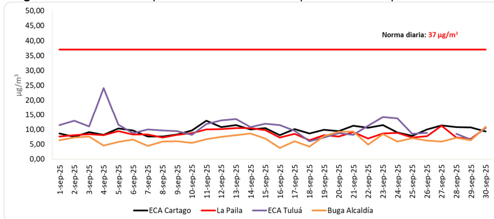
Figura 2. Concentración promedio diaria de PM2.5 por estación. Septiembre de 2025.
