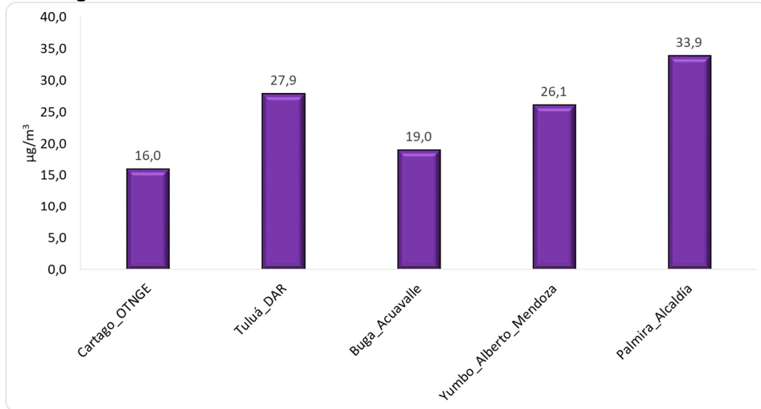
Figura 6. Media móvil octohoraria de O 3 . Cuarto trimestre de 2025
