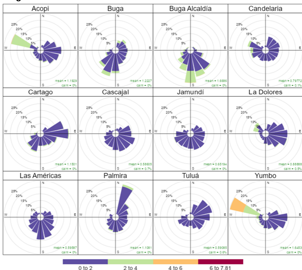
Figura 15. Rosa de los Vientos SVCA de la CVC. Cuarto trimestre de 2025
