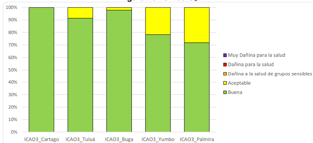
Figura 23. ICA de O 3 .
