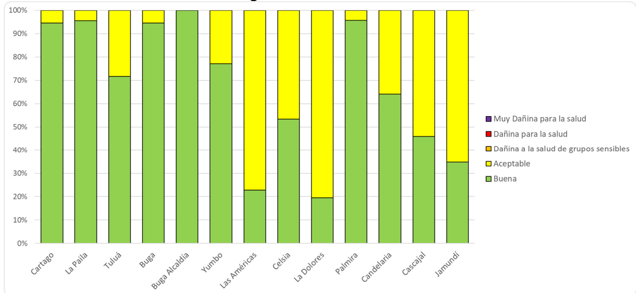
Figura 21. ICA de PM2.5.
