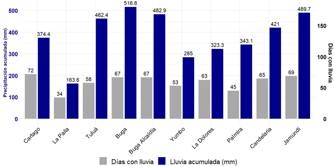
Figura 18. Precipitación acumulada. Cuarto trimestre de 2025
