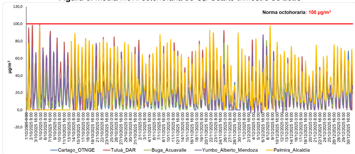
Figura 6. Media móvil octohoraria de O 3 . Cuarto trimestre de 2025
