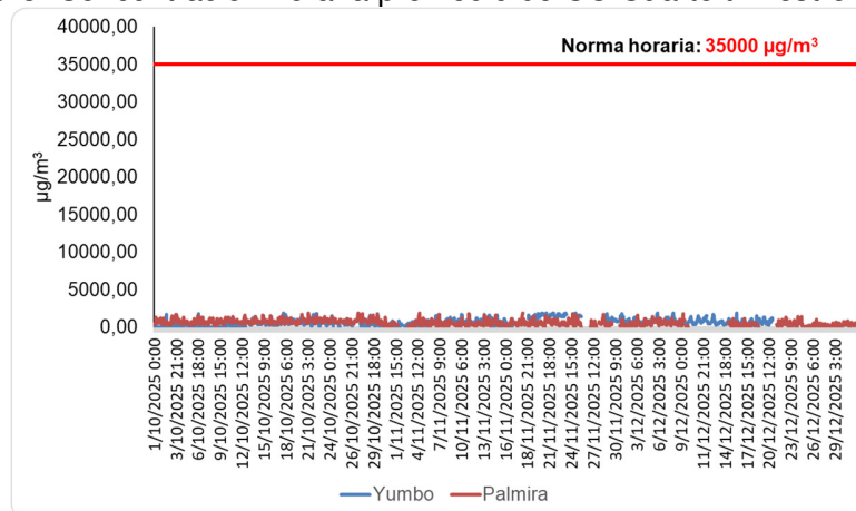
Figura 8. Concentración horaria promedio de CO Cuarto trimestre de 2025
