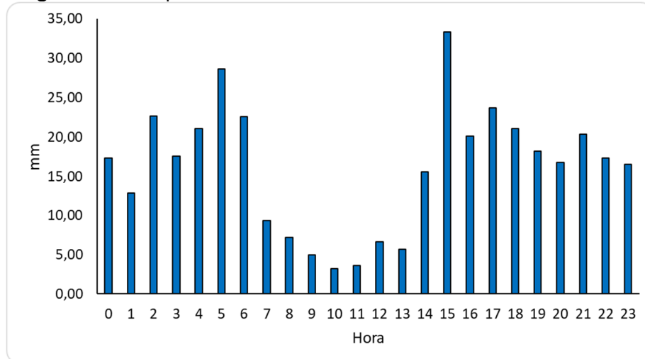
Figura 19. Precipitación acumulada horaria. Cuarto trimestre de 2025
