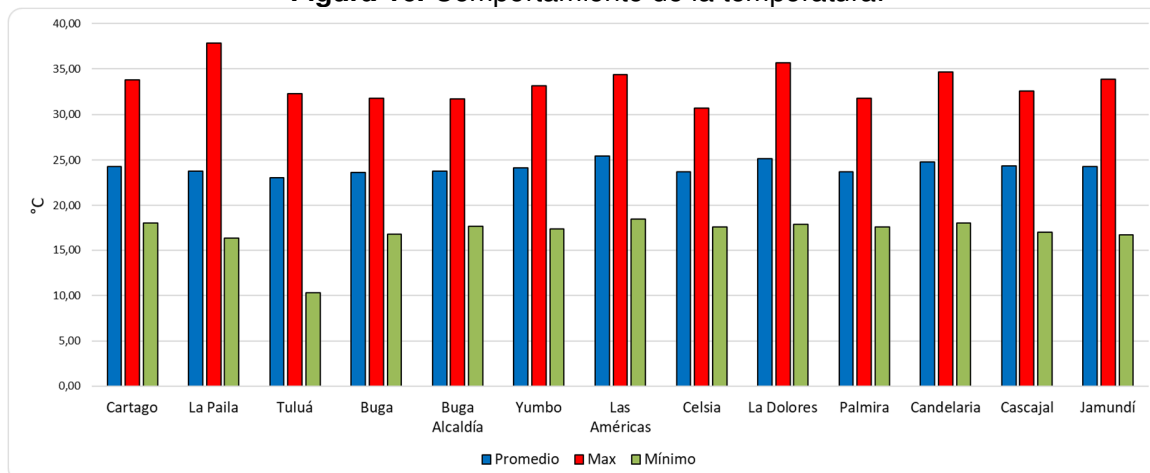
Figura 16. Comportamiento de la temperatura.
