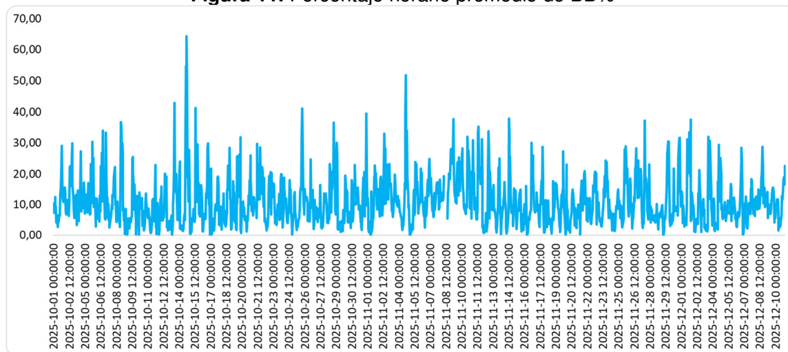
Figura 11. Porcentaje horario promedio de BB%
