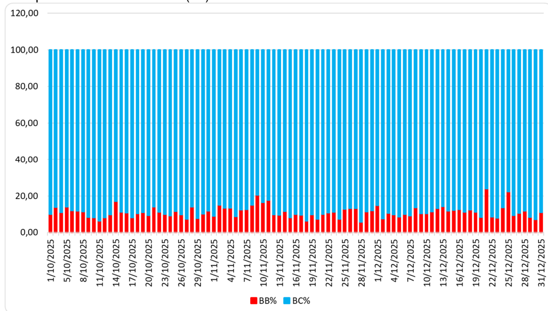
Figura 14. Serie temporal porcentaje de quema Black Carbón de combustibles fósiles BC%(ff) vs. Black Carbón de quema de biomasa BB%(bb) – Cuarto trimestre de 2025.
