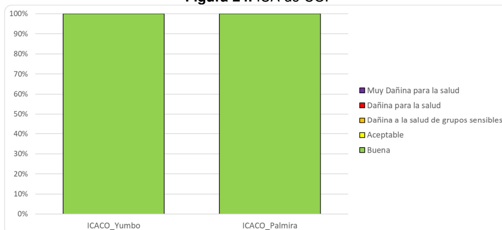
Figura 24. ICA de CO.
