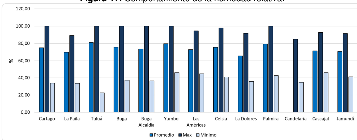
Figura 17. Comportamiento de la humedad relativa.
