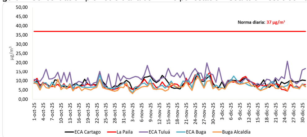
Figura 2. Concentración promedio diaria de PM2.5 por estación. Cuarto trimestre de 2025.
