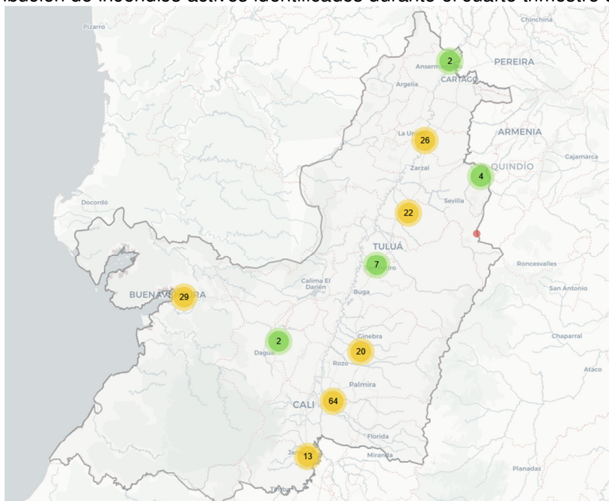
Figura 13. Distribución de incendios activos identificados durante el cuarto trimestre de 2025.
