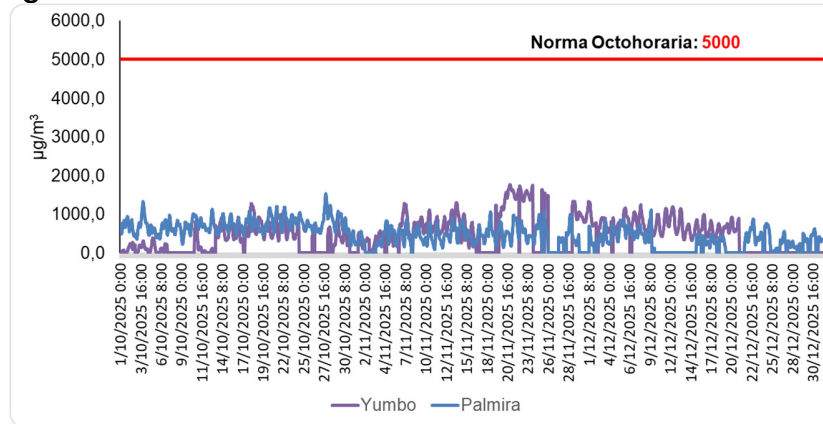
Figura 7. Media móvil octohoraria de CO. Cuarto trimestre de 2025
