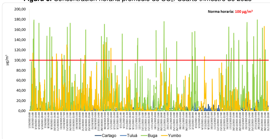
Figura 3. Concentración horaria promedio de SO 2 . Cuarto trimestre de 2025
