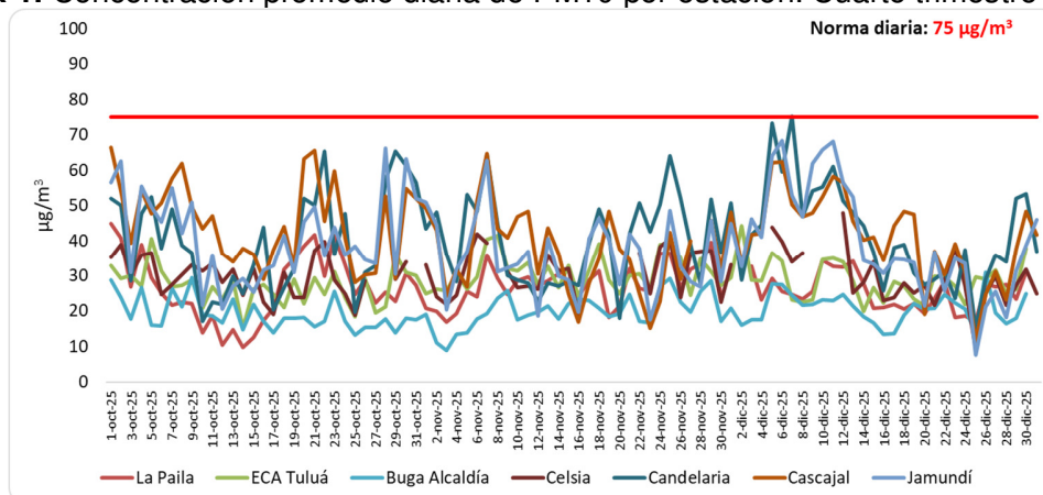
Figura 1. Concentración promedio diaria de PM10 por estación. Cuarto trimestre de 2025
