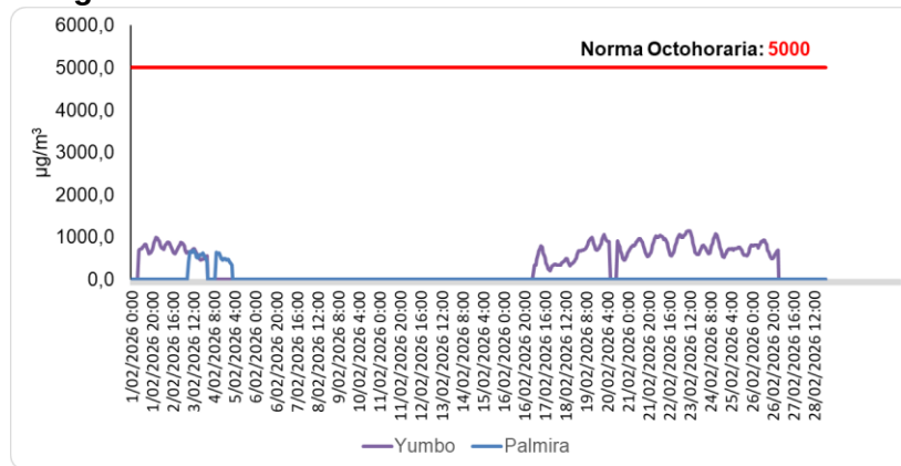
Figura 7. Media móvil octohoraria de CO. febrero de 2026
