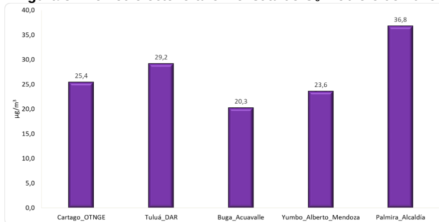
Figura 5. Promedio octohorario mensual de O 3 . Febrero de 2026
