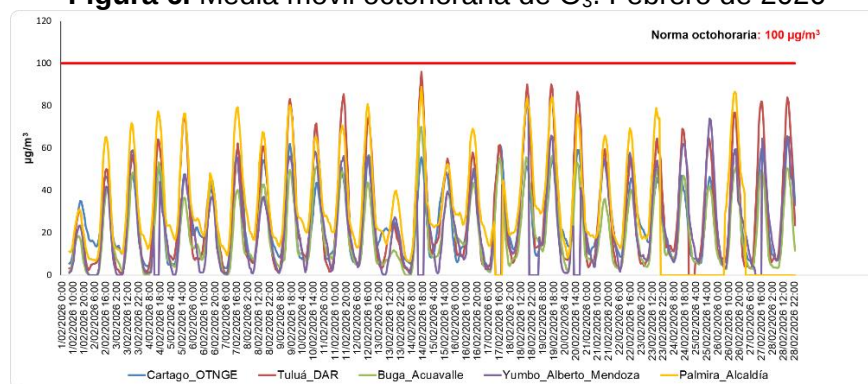
Figura 6. Media móvil octohoraria de O 3 . Febrero de 2026
