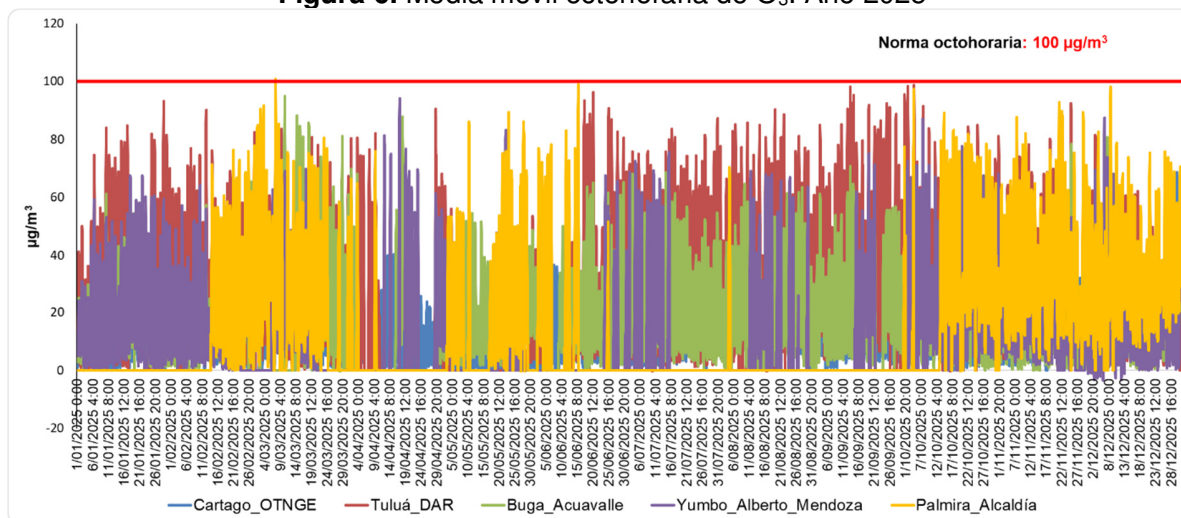
Figura 6. Media móvil octohoraria de O 3 . Año 2025
