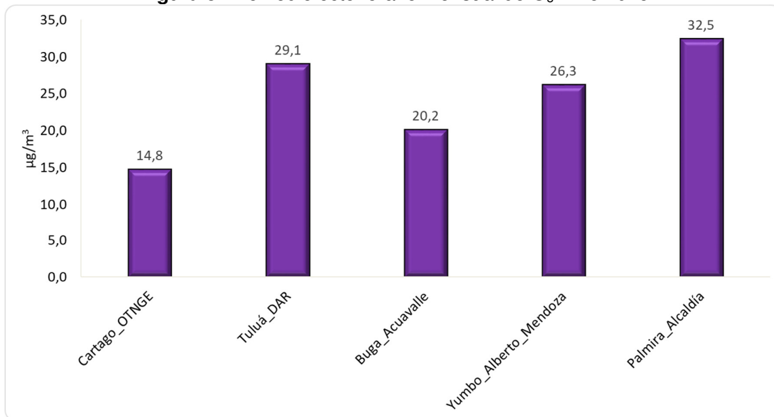
Figura 5. Promedio octohorario mensual de O 3 . Año 2025
