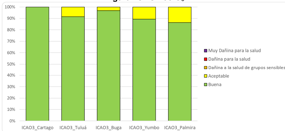
Figura 23. ICA de O 3 .
