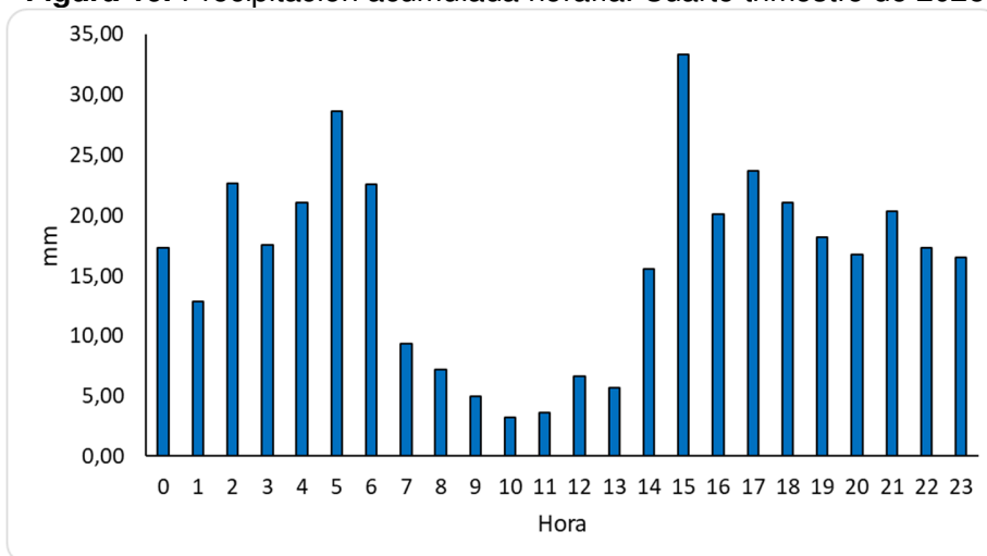
Figura 19. Precipitación acumulada horaria. Cuarto trimestre de 2025
