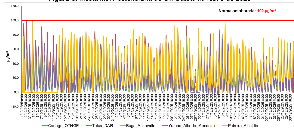
Figura 6. Media móvil octohoraria de O 3 . Cuarto trimestre de 2025
