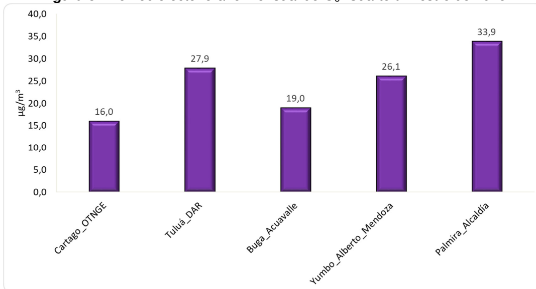
Figura 5. Promedio octohorario mensual de O 3 . Cuarto trimestre de 2025
