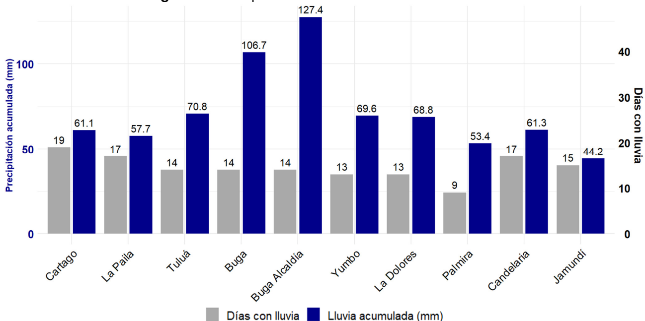
Figura 18. Precipitación acumulada. Diciembre de 2025
