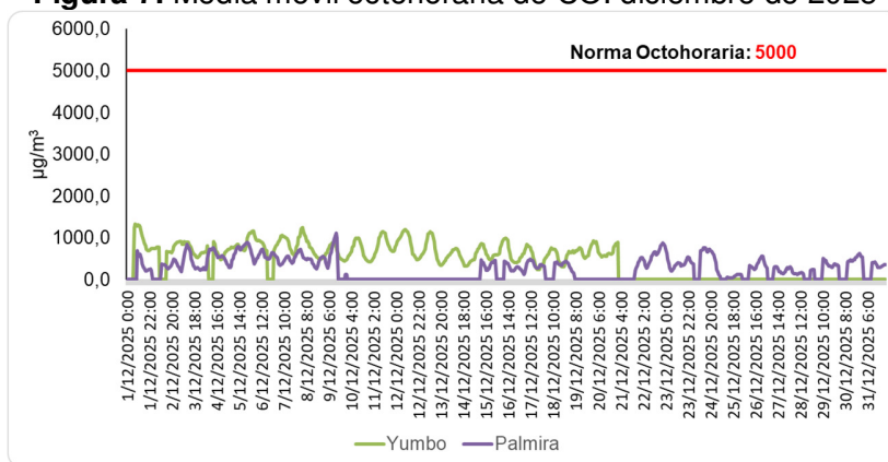
Figura 7. Media móvil octohoraria de CO. diciembre de 2025
