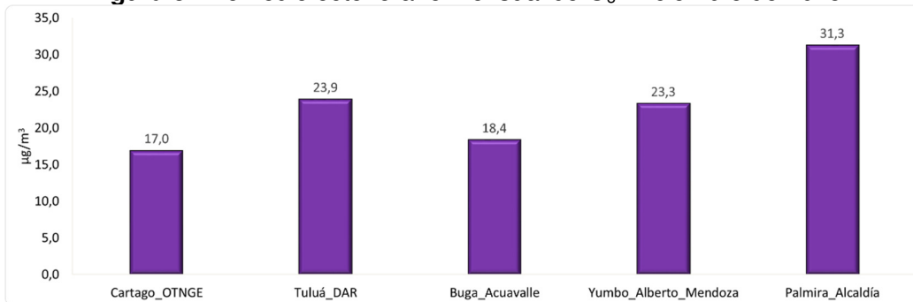
Figura 5. Promedio octohorario mensual de O 3 . Diciembre de 2025
