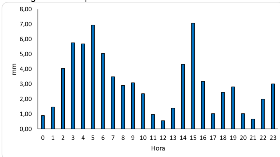
Figura 19. Precipitación acumulada horaria. Diciembre de 2025
