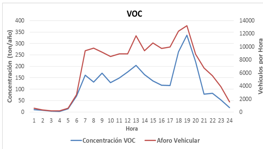
Figura 6.12 Emisión horaria VOC por fuentes móviles vs aforo vehicular – Buga. Fuente: K2 Ingeniería S.A.S (estudio actual)
