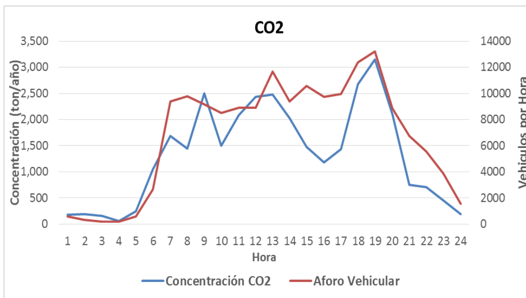
Figura 6.18 Emisión horaria CO 2 por fuentes móviles vs aforo vehicular – Buga. Fuente: K2 Ingeniería S.A.S (estudio actual)
