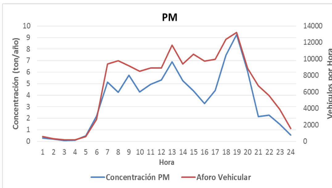
Figura 6.16 Emisión horaria PM por fuentes móviles vs aforo vehicular – Buga. Fuente: K2 Ingeniería S.A.S (estudio actual)
