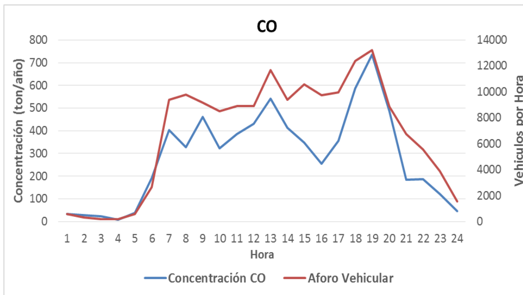
Figura 6.11 Emisión horaria CO por fuentes móviles vs aforo vehicular – Buga. Fuente: K2 Ingeniería S.A.S (estudio actual)
