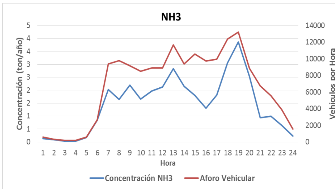
Figura 6.17 Emisión horaria NH3 por fuentes móviles vs aforo vehicular – Buga. Fuente: K2 Ingeniería S.A.S (estudio actual)
